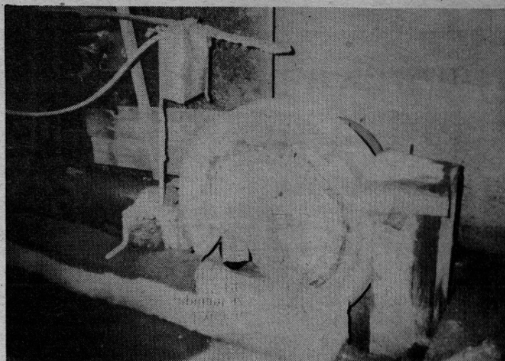
Le redki primerki takšnega brusa za orodja so še v uporabi. Orodni kovač Krajnc v Konjskem vrhu še vedno brusi nanj.
