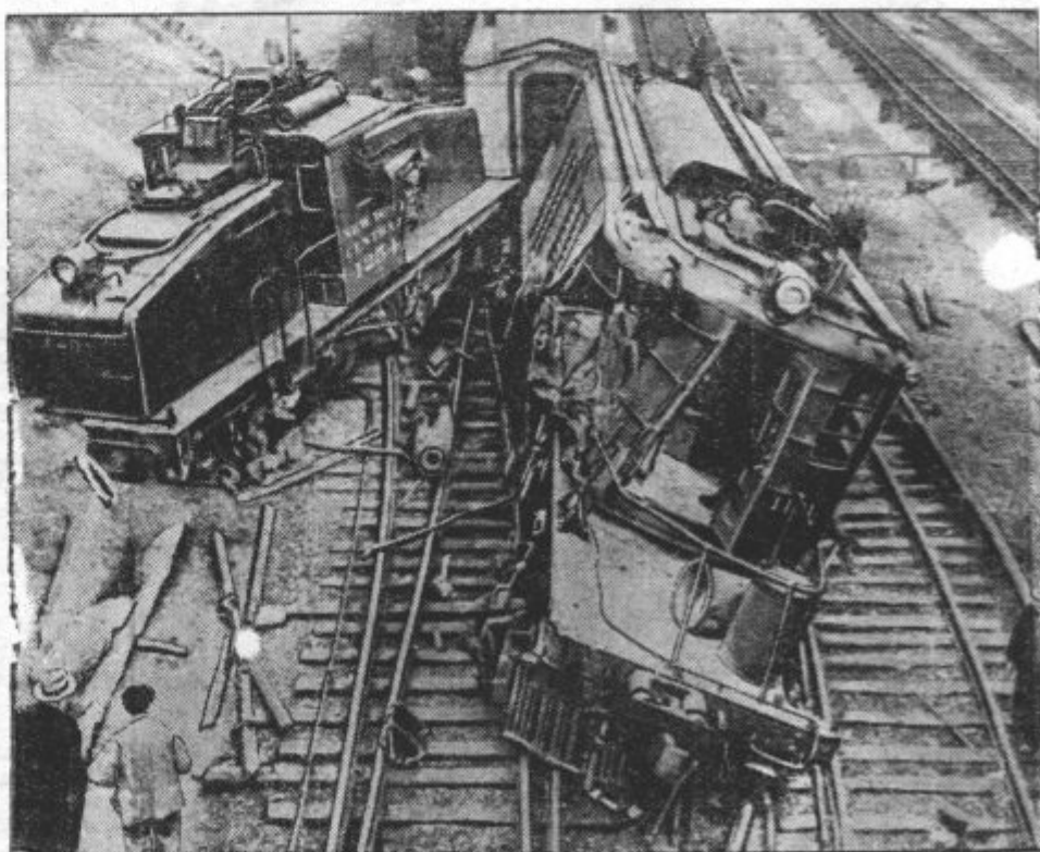
Trčenje dveh brzovoznih lokomotiv
