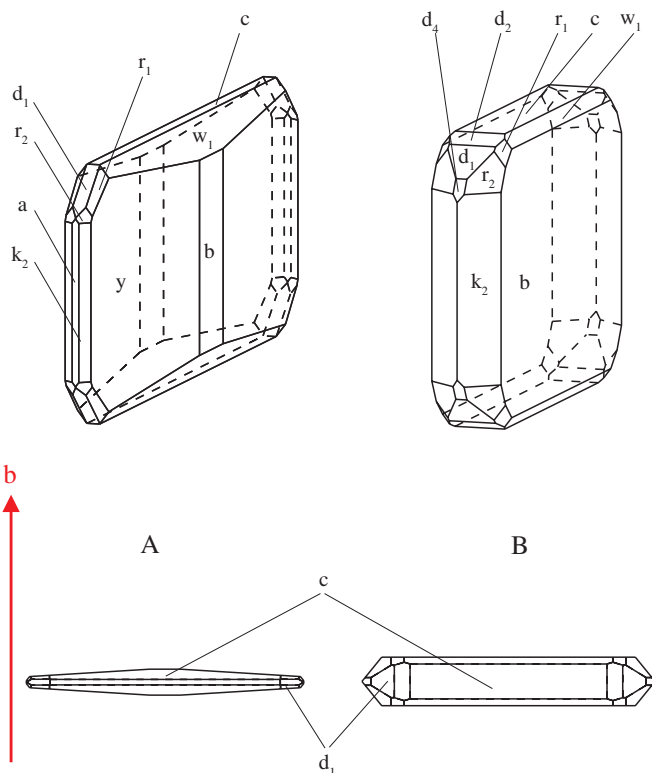
Ploskovno bogat kristal barita prve generacije (A) in njegova projekcija na ravnino (001). Tipičen kristal barita druge generacije (B) in njegova (001) projekcija. Rdeča puščica označuje smer b-osi v (001) projekciji. Risbe: Mirjan Žorž
