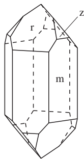
Kristal kremen a omejujejo le ploskve prizme m\{100\} ter pozitivnega r\{101\} in negativnega z\{011\} romboedra. Risba: Mirjan Žorž
