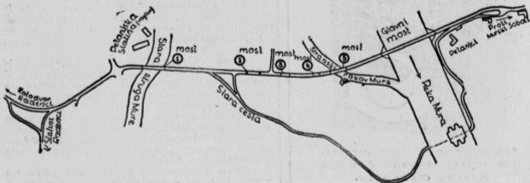
Skica kaže preložitev ceste pri Petanjcih in lego glavnega mostu in inundacijskih mostov.
