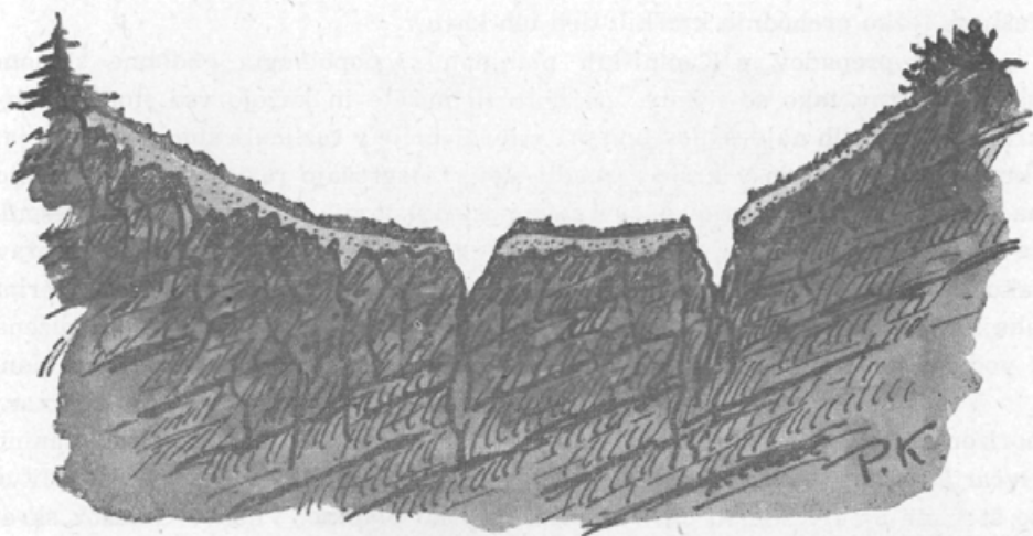
Vrtača, pokrita s prstjo in rušo, v nji dve mali ponikvi.
