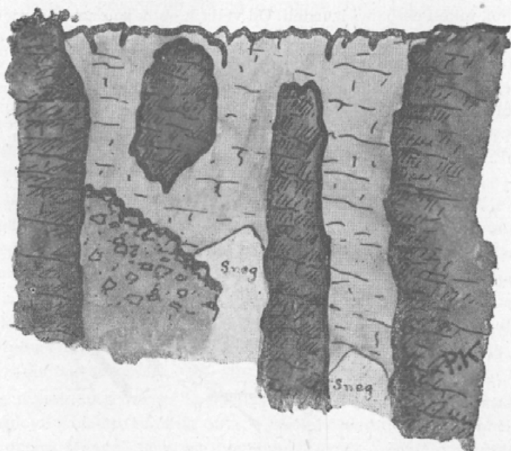
Skupina treh pre- padov na sedlu med Velikim vrhom in Crnim vrhom nad Moličko planino.
