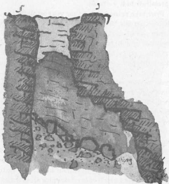
Prepad Mala vetrnica na Veliki planini. V dnu sneg in ledene sveče poleti.
