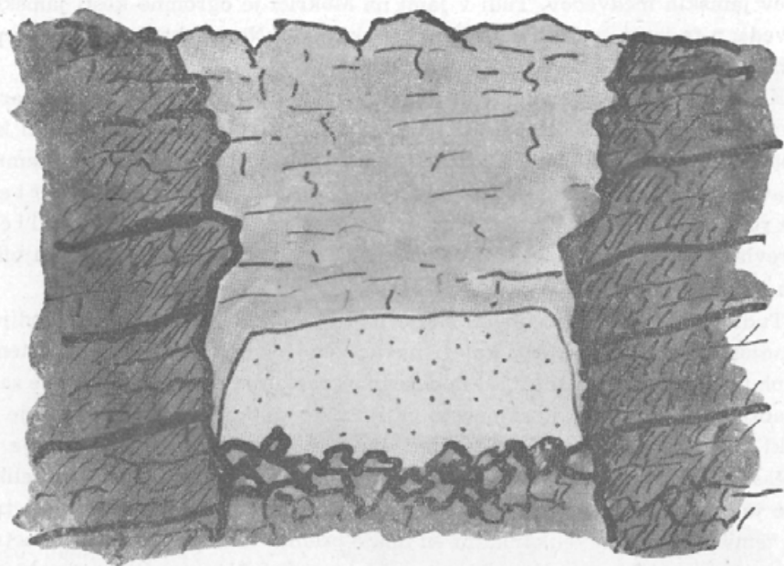
Kotlič v visokogorskem krasu s snegom. Pozno poleti.
