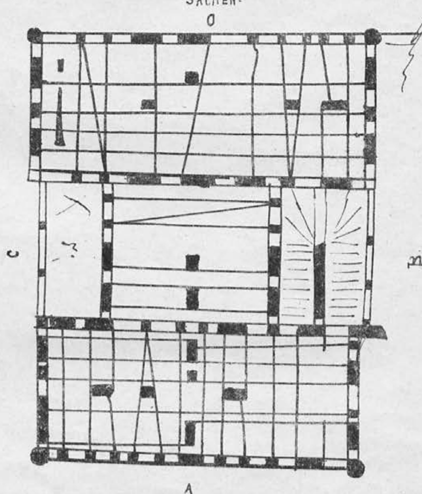
PLÄNE VON VERSCHIEDENEN HÄUSERN IN POMP. E. I. UND HERUKULANUM U. S. W.
