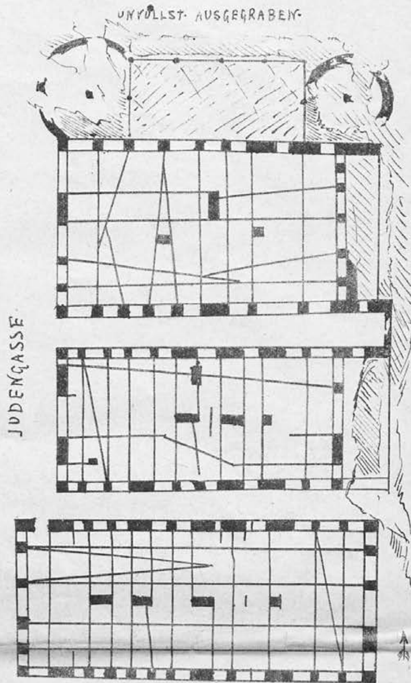
MARKTHALLE [BASILIKA] FÜR DEN KLEINVERSCHLEISS VON VERSCH. SACHEN.
