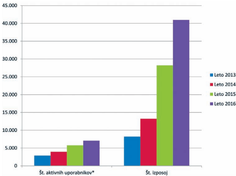
Podatki o številu aktivnih uporabnikov in številu izposojenih e-knjig na uporabnika preko Biblosa med letoma 2013 in 2016. (Opomba: *uporabniki, ki si na mesec izposodijo vsaj eno e-knjigo.)
