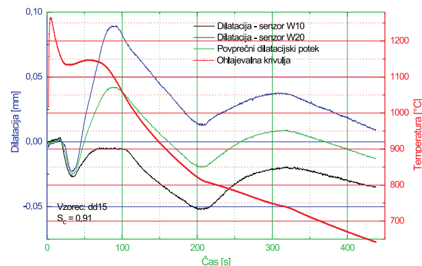
Slika 4: Dilatometrijske krivulje in ohlajevalna krivulja podevtske sive litine s kroglastim grafitom (dd15); S_c je stopnja nasičenja
