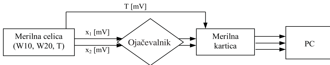
Slika 2: Shema dilatometra
