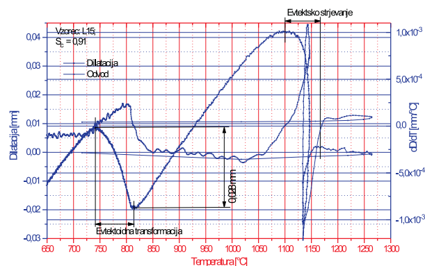
Slika 5: Dilatacija feritne sive litine s kroglastim grafitom v odvisnosti od temperature in odvod dilatacijske krivulje (L15)
