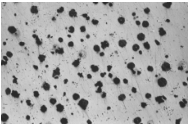
Slika 8: Grafit v nemodificirani sivi litini s kroglastim grafitom (L37), S_C = 0,92 ; a) polirano, povečava 100-krat, grafitni noduli, b) jedkano z nitalom, povečava 100-krat, mikrostruktura matrice pretežno perlitne sive litine s kroglastim grafitom
