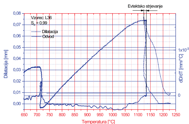
Slika 9: Dilatacija sive litine z lamelnim grafitom v odvisnosti od temperature in odvod dilatacijske krivulje (L36)
