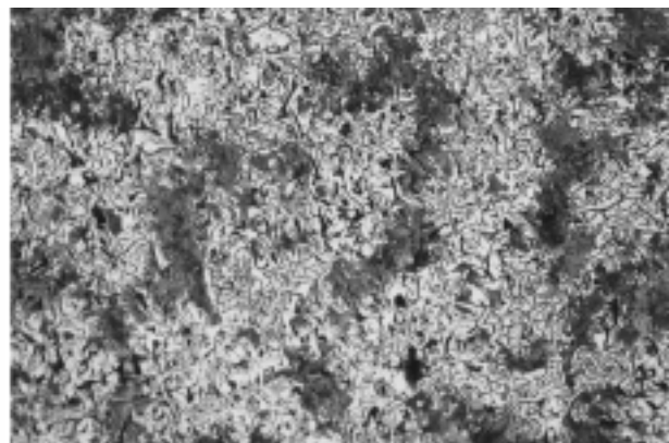
Slika 10: Grafit v nemodificirani sivi litini z lamelnim grafitom (L36), S_C = 0,99 ; a) polirano, povečava 100-krat, lamelni in rahlo vermikularni grafit, b) jedkano z nitalom, povečava 100-krat, mikrostruktura matrice sive litine z lamelnim grafitom, ob grafitu ferit in perlit
