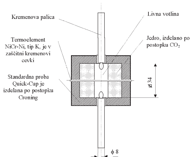
Slika 3: Shema merilne celice
