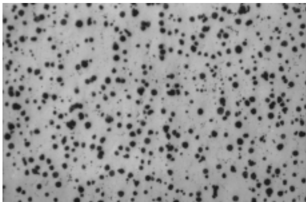
Slika 6: Grafit v sivi litini s kroglastim grafitom (L15), S_C = 0,91 ; a) polirano, povečava 100-krat, grafitni noduli, b) jedkano z nitalom, povečava 100-krat, mikrostruktura matrice feritne sive litine s kroglastim grafitom, ob grafitu ferit, perlit
