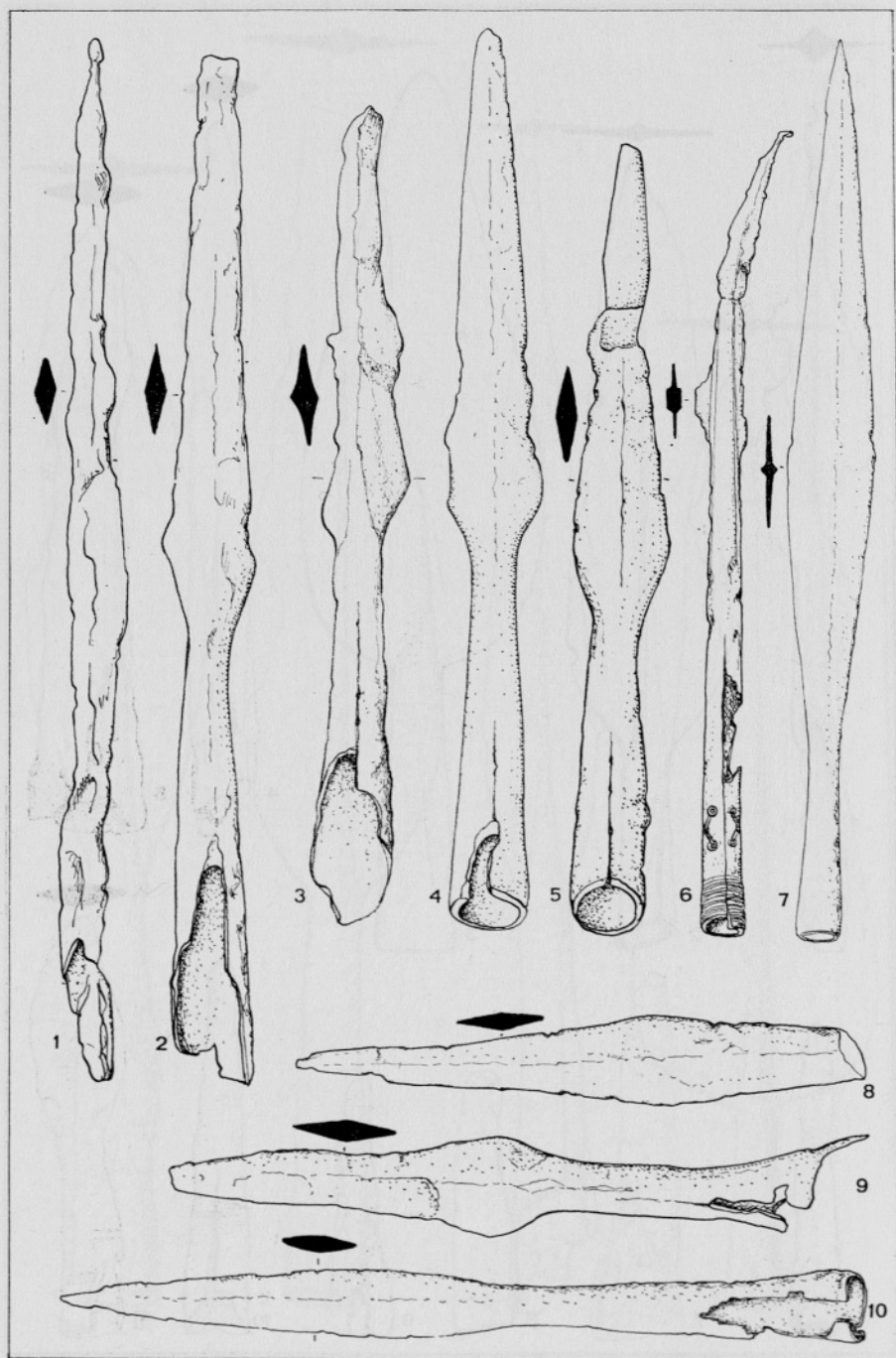
Valična vas. Železo — Eisen. 1—5, 8—10 = 1/2, 6, 7 = 1/4
