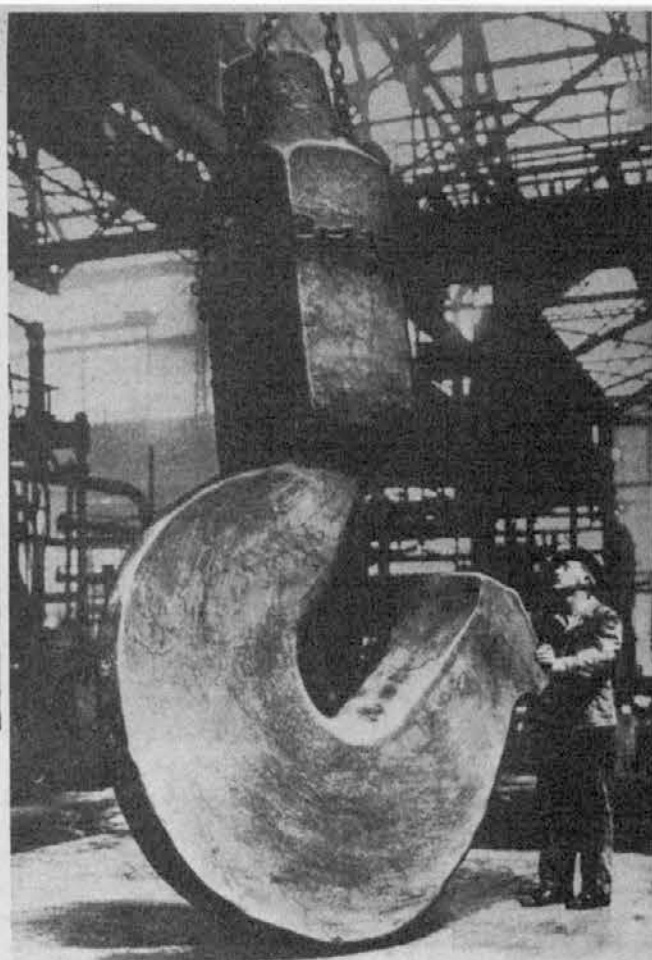
Na desni: 7000 kg težka železna kljuka, ki so jo izdelali v Nemčiji za enega največjih ladjedelniških žerjavov.
