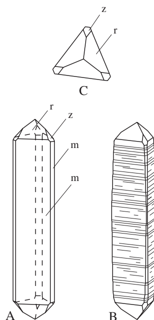
Kristali kremena – ametista iz kamnoloma Leva. Idealiziran kristal (A) in njegova terminacija (C) s ploskvami prizme m\{100\} ter pozitivnega r\{101\} in negativnega romboedra z\{011\} . Realni kristali (B) so trebušasti in narebreni na ploskvah prizme m\{100\} . Risbe: Mirjan Žorž
