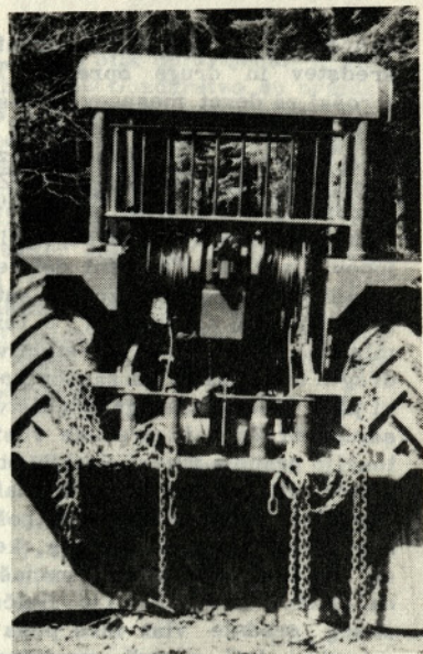
Ferguson adaptiran v gozdarski traktor s švedskim vitlom IG-LAND. Foto: I. V.
