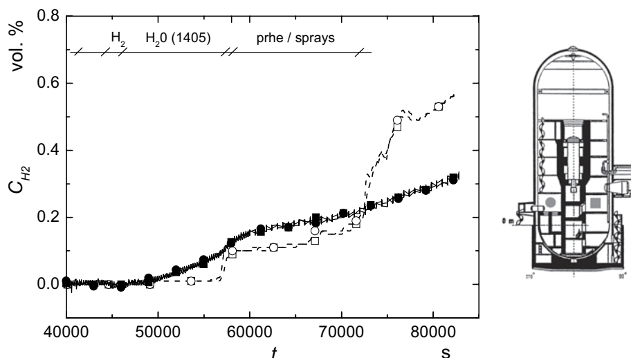
Sl. 14. Koncentracija vodika v spodnjem delu stopnišč (polne črte: meritve, črtkane črte: simulacija, t : čas, C : prostorninska koncentracija)
