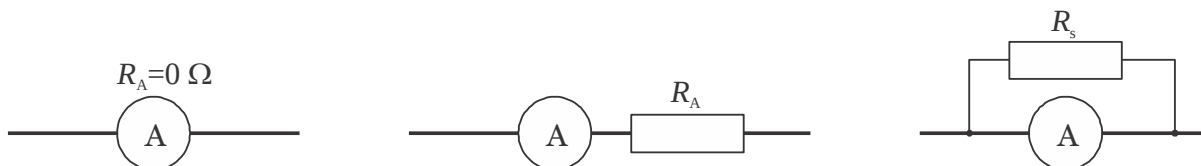
Slika 23-20: idealni ampermeter (levo), ampermeter z notranjo upornostjo (sredina), razširitev merilnega območja ampermetra s souporom (desno)
