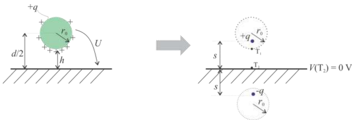
Slika 15-2: Naelektren valj nad zemljo analiziramo s pomočjo zrcaljenja ekscentrično postavljenega premega naboja in njegovega zrcalnega naboja.
