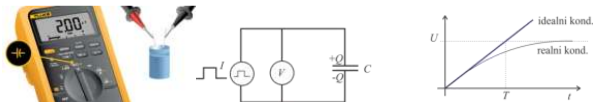
Slika 16-2: Univerzalni inštrumenti običajno omogočajo tudi merjenje kapacitivnosti. Pri tem skozi kondenzator pošljejo določen tok in ga s tem elektrijo. Kapacitivnost je sorazmerna času elektrenja in obratno sorazmerna napetosti.
