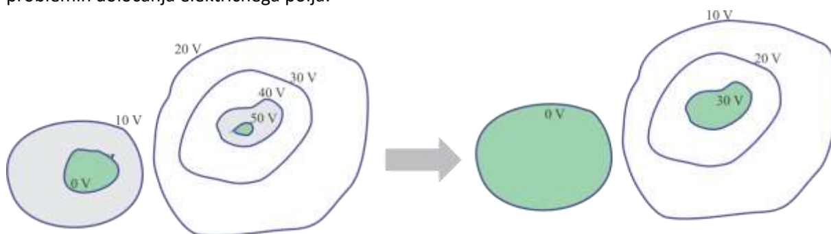
Slika 14-1: Levo razmere pred okovinjenjem (s sivo površino je nakazano področje okovinjenja). Desno: razmere po okovinjenju. Razmere med ekvipotencialkama se ne spremenijo, če je le napetostna razlika med okovinjenima ekvipotencialkama enaka kot je bila predhodno pred okovinjenjem.
