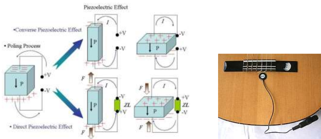
Slika 17-7: Levo: Piezelektrični material polariziramo tako, da ga izpostavimo velikemu električnemu polju. Pri mehanski obremenitvi deluje v generatorskem principu – na površini se pojavi vezan naboj zaradi spremembe polarizacije. Če pa nanj priključimo napetost, se bo pojavila mehanska sila in s tem deformacija piezelektrika (stisk ali raztezek). Desno: piezelektrik kot senzorski element za zaznavanje tresljajev.
