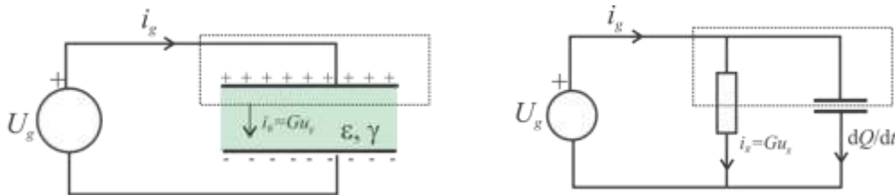
Slika 20-9: Levo: realni kondenzator priključen na vir napetosti U_g . Desno: preprost model realnega kondenzatorja upošteva njegovo notranjo upornost.
