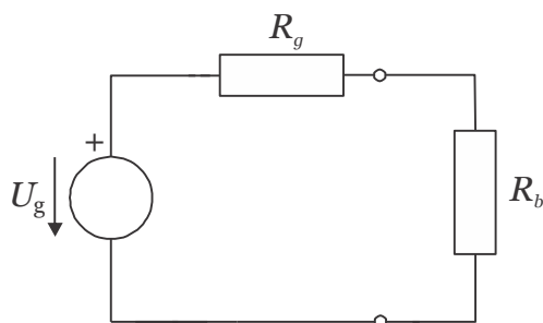
Slika 23-25: Moč na bremenu R_b , ki je priključen na realni napetostni vir. Levo: breme na realnem napetostnem viru, desno: prikaz moči na bremenu v odvisnosti od R_b .
