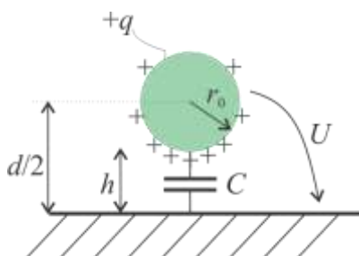
Slika 16-3: Prevodni valj nad zemljo.
