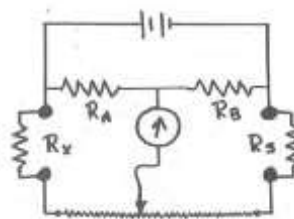
Slika: Kirchhoffov mostič temelji na gibljivem (drsnem) kontaktu in omogoča merjenje majhnih upornosti. (Vir: Error! Reference source not found. in Error! Reference source not found.)
