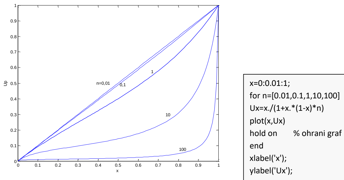
Slika 23-14: U_b za različna razmerja n = R / R_b . n = 0,01, 0,1, 1, 10, 100 . Večjo linearnost se doseže pri n \ll 1 , torej tedaj, ko je bremenska upornost dosti večja od upornosti uporabnega delilnika.
