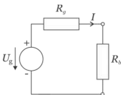
Slika 23-3: Levo: shema realnega napetostnega vira s priključenim bremenom. Desno: karakteristika realnega napetostnega vira in karakteristika priključenega bremenja. V presečišču dobimo delovno točko.
