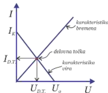
Slika 23-3: Levo: shema realnega napetostnega vira s priključenim bremenom. Desno: karakteristika realnega napetostnega vira in karakteristika priključenega bremenja. V presečišču dobimo delovno točko.
