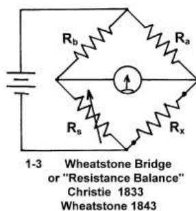
Slika: Ena osnovnih izvedenk Wheatstonovega mostiča, ki ga je sam imenoval diferencialni merilnik upornosti. (Hampden-Sydney College, Virginia), na desni »modernejša« izvedba. (Greenslade collection) Vir: Error! Reference source not found. in Error! Reference source not found..
