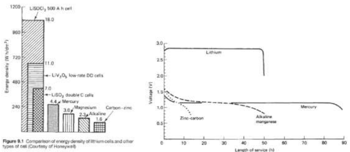
Slika 21-9: Levo: primerjava prednosti litijevih baterij pred ostalimi glede na gostoto energije. Desno: napetostne karakteristike v(t) raznih tipov baterij. Vir: T.R. Crompton: Battery reference book, Newnes, 2000.
