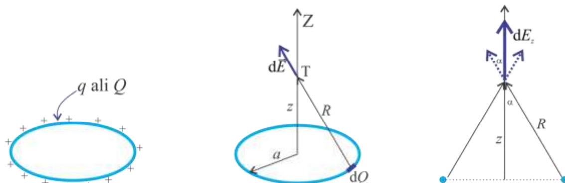
Slika 6-8: Prikazi za izračun polja v osi enakomerno naelektrenega obroča.
