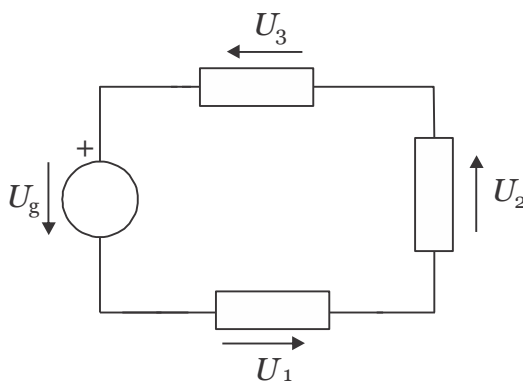
Slika 22-2: Idealni napetostni generator in zaporedno vezani upori v zanki. Po 2. Kirchhoffovem zakonu mora veljati, da je vsota vseh padcev napetosti v zanki enaka nič
