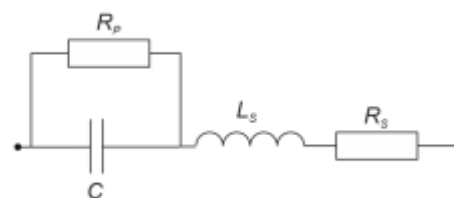
Slika 19-6: Nadomestna shema realnega kondenzatorja.
