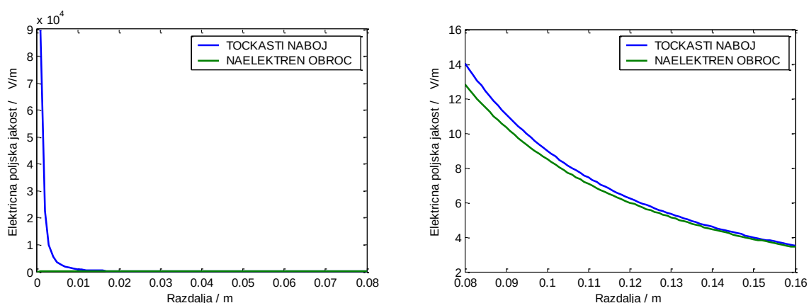
Slika 6-12: Primerjava med poljem v oddaljenosti od točkastega naboja in v osi naelektrenega obroča. Oba imata enako velik naboaj (0,1 nc, polmer prstana je 2 cm). Levo: polje v bližini obroča. Desno: polje v
