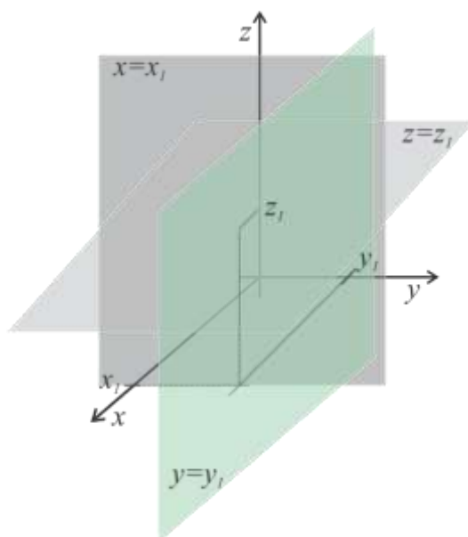
Slika 5-1: Kartezični koordinatni sistem.
