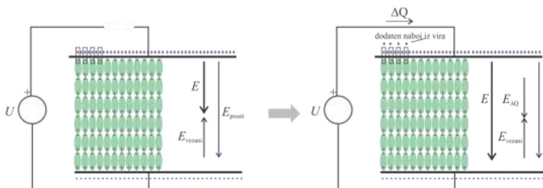
Slika 17-2: Ker se polje znotraj dielektrika zmanjša zaradi polarizacije nabojev v dielektriku, mora za vzpostavitev priključene napetosti iz vira priteči dodaten naboj. Levo: naelektren kondenzator brez priključene napetosti. Desno: kondenzator ob priključeni napetosti.
