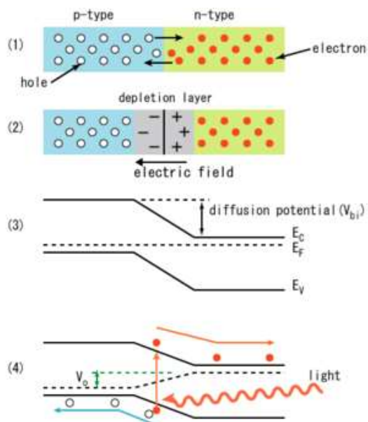
Slika 21-10: Levo: Sončna celica sestavljena iz polprevodniškega pn spoja. Na površini je antirefleksni sloj, ki povečuje absorpcijo svetlobne energije. Desno: ob stiku p in n tipa polprevodnika pride do prerazporeditve nabojev in vgrajenega električnega polja. Sončni žarki imajo dovolj veliko energijo, da povzročijo generacijo para elektron-vrzel. Če se to zgodi v (osiromašenem) področju električnega polja, se naboja ločita, presežki pa povzročijo tok v sklenjenem tokokrogu.
