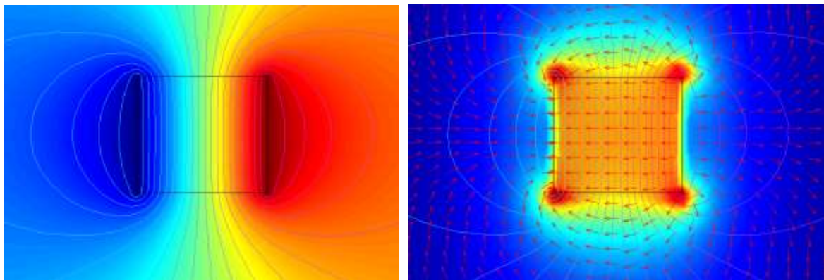
Slika 9-10: Levo: ekvipotencialne ploskve med in v okolici dveh nasprotno naelektrenih ravnih plošč. Ugotovimo, da so med ploščama ekvipotencialne ploskve enakomerno razmaknjene, v okolici pa ne (bolj goste so ob robovih elektrod). Desno: vektorji električne poljske jakosti skupaj z ekvipotencialnimi ploskvami in velikostjo električne poljske jakosti (večje polje bolj rdeča barva). Za lažje opazovanje so vektorji polja prikazani enako veliki neodvisno od velikosti polja.
