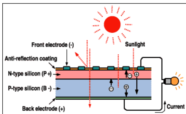
Slika 21-10: Levo: Sončna celica sestavljena iz polprevodniškega pn spoja. Na površini je antirefleksni sloj, ki povečuje absorpcijo svetlobne energije. Desno: ob stiku p in n tipa polprevodnika pride do prerazporeditve nabojev in vgrajenega električnega polja. Sončni žarki imajo dovolj veliko energijo, da povzročijo generacijo para elektron-vrzel. Če se to zgodi v (osiromašenem) področju električnega polja, se naboja ločita, presežki pa povzročijo tok v sklenjenem tokokrogu.
