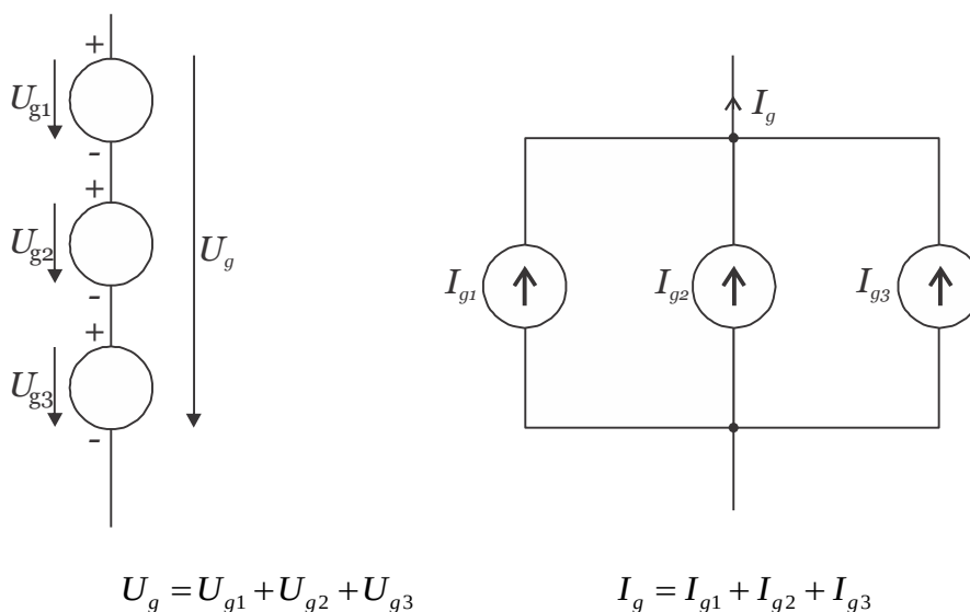
Slika 23-6: Zaprordna vezava napetostnih virov in vzporedna vezava tokovnih virov.
