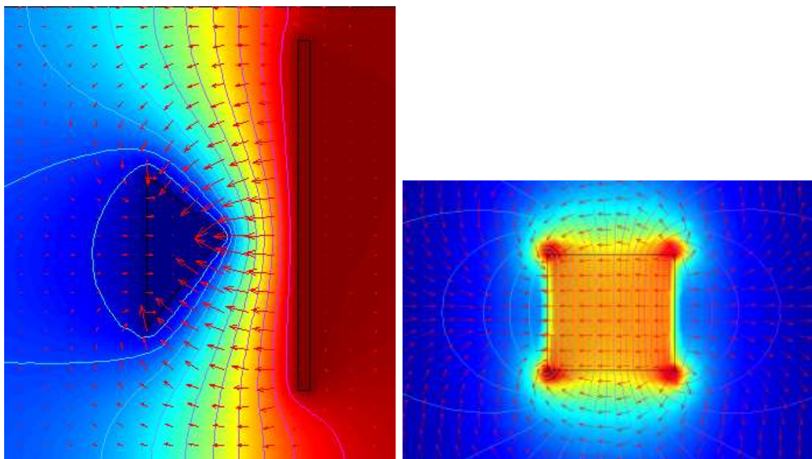
Slika 11-3: Električna poljska jakost kaže smer in hitrost upadanja potenciala. Primera polja klinaste elektrode ob ravni elektrodi in polja med ravnima ploščama. Na levi sliki so poleg vektorjev polja prikazane še ekvipotencialne ravnine ter potencial v barvni lestvici. Na desni sliki pa so zaradi lažjega opazovanja vektorji polja normirani, velikost polja pa prikazuje barvna lestvica. Poleg tega so prikazane ekvipotencialne ravnine.
