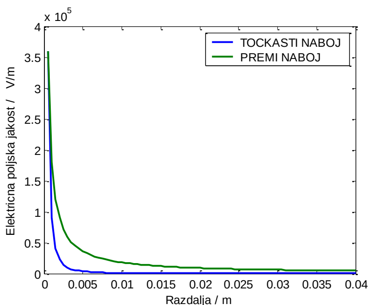
Slika 6-13: primerjava med poljem točkastega (modra črta) in premga naboja (zeleni črta). Polje točkastega naboja upada s kvadratom razdalje (1/r 2 ), polje premga pa z razdaljo (1/r).
