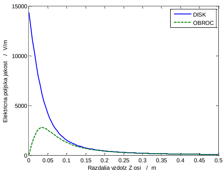
Slika 6-10: Primerjava polj vzdolž osi Z naelektrenega obroča (črtkana zelena črta) in naelektrenega diska (polna modra črta).
