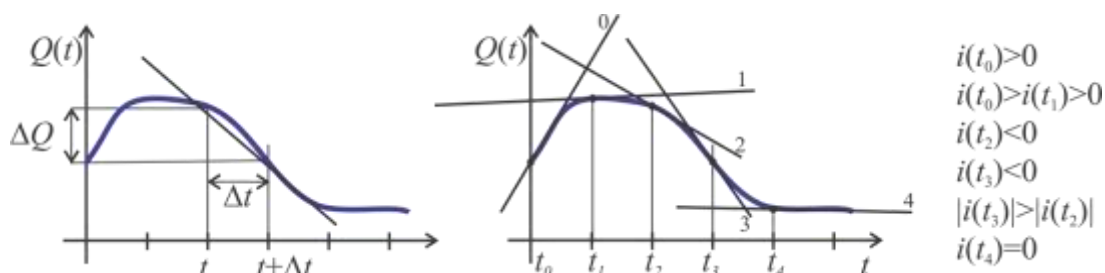
Slika 1-3: Električni tok je enak hitrosti spreminjanja množine naboja na telesu. Z manjšanjem časovne spremembe med dvema odčitkoma ugotovimo, da določimo tok iz naklona tangente na Q - t krivulji ob želenem času. Večji naklon pomeni večji tok, smer naklona pa smer toka.
