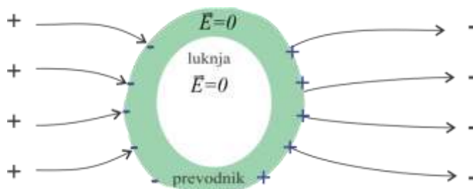
Slika 10-4: Polje znotraj luknje v prevodniku je enako nič. Tako strukturo pogosto imenujemo Faradayeva kletka in je popularen rekvizit za prikazovanju električnih eksperimentov. Uspešno ščiti notranjost kletke pred zunanjim elektrostatičnim poljem pa tudi dinamičnem (elektromagnetnim), če je le valovna dolžina elektromagnetnega polja večja od širine odprtin. Ne more pa Faradayeva kletka ščititi pred magnetostatičnim poljem ali magnetnim poljem nizkih frekvenc. Več o tem v drugem semestru. Več: http://tesladowndunder.com/
