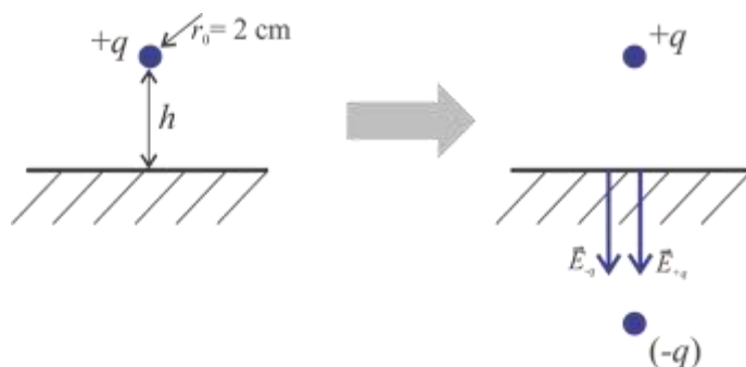
Slika 15-3: Daljnovodna vrv na zemljo: izračun polja in potenciala poteka s pomočjo zrcaljenja premega naboja preko površine zemlje.
