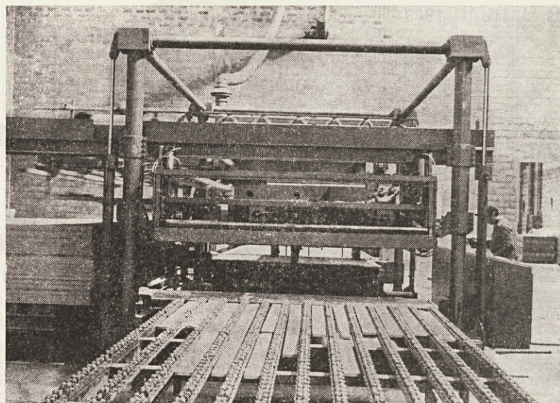
Razrez ivernih plošč v TOZD IVERKA
