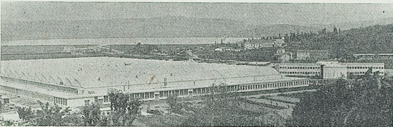
Pogled na tovarno motornih koles TOMOS v Kopru, kakršna je še danes. Zakaj jutri bo že drugačna, še večja in sodobnejša, saj bo razen motornih koles izdelovala tudi štirikolesna motorna vozila. Ta objekt je po pravici naš ponos, saj je živ zgled naše vztrajnosti in vere v lepše življenje v socialistični Jugoslaviji, živ zgled, kako se v naši domovini lahko uveljavijo zdrave pobude sposobnih organizatorjev proizvodnje in živ zgled, kako zlahka se naši bistri delovni ljudje prilagodijo in priučijo novemu, do večerj morda še neznanemu delu. Pravkar slavi TOMOS še poseben praznik: kljub nasprotnim prerokovanjem je uspela tovarna še pred koncem leta izpolniti plan podjetja in se tako popolnoma uveljaviti kot enakopravna gospodarska organizacija vsem jugoslovanskim podjetjem, čeprav njena izgradnja še ni povsem končana
