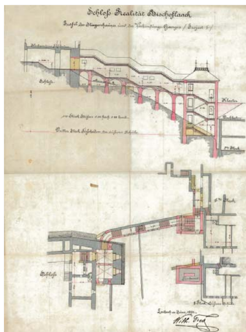
Sl. 14: Tretji list načrta Loškega gradu arhitekta Wiljema Trea, kjer je vidna ena od nerealiziranih variant pokritega stopnišča, ki je povezovalo grad s samostanom v mestu. (hrani Loški muzej)
