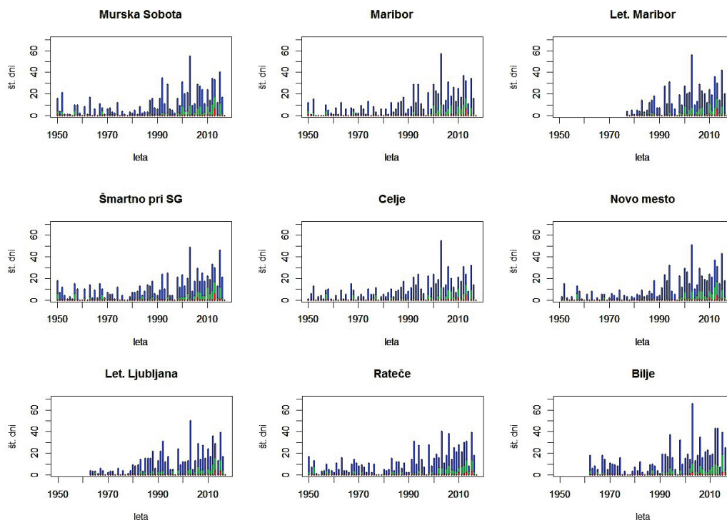
Slika 7. Prikaz števila dni na leto, ko so izpolnjeni pogoji za vročinski val (modri stolpci), ko bi lahko imeli nevarne razmere (zeleni stolpci) in ko so bile razmere zelo nevarne (rdeči stolpci). Po vrsti so prikazani rezultati za postaje Murska Sobota, Maribor, Letališče E. Rusjana Maribor, Šmartno pri Slovenj Gradcu, Celje, Novo mesto, Kočevje, Postojna, Ljubljana, Letališče J. Pučnika Ljubljana, Rateče in Bilje.
