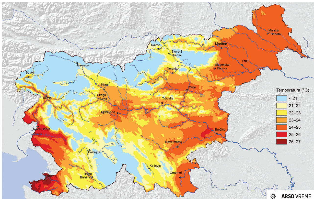
Slika 4. Prostorska porazdelitev dnevne povprečne temperature zraka pri 96. centilu v obdobju 2006–2015 (DPT96).
