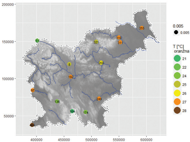
Slika 3. Vrednosti ocenjene povprečne dnevne temperature za oranžno stopnjo ogroženosti na posameznih obravnavanih postajah po Sloveniji. Številke na obarvanih krogih na zemljevidu predstavljajo številko postaje.
