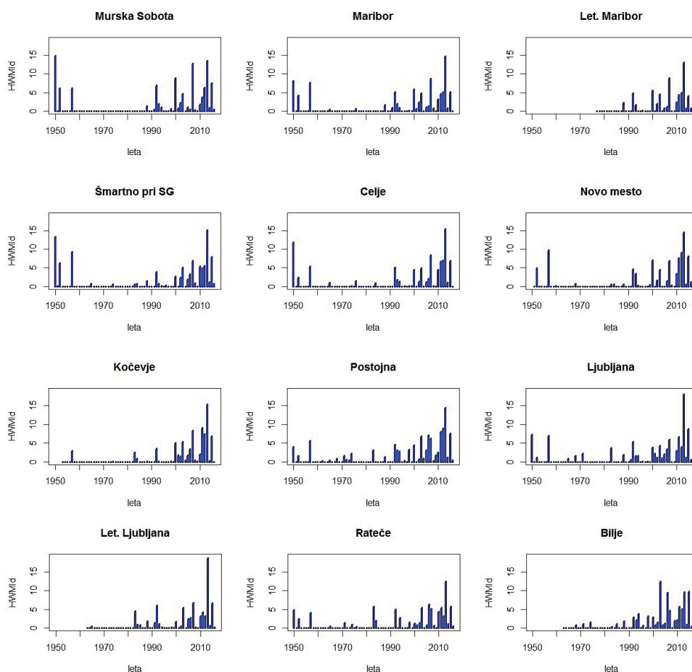
Slika 9. Vrednosti kazalca HWMId v posameznem letu, kar predstavlja najmočnejši vročinski val v tistem letu glede na trajanje in glede na magnitudo. Po vrsti so predstavljene vrednosti na postajah Murska Sobota, Maribor, Letališče E. Rusjana Maribor, Šmartno pri Slovenj Gradcu, Celje, Novo mesto, Kočevje, Postojna, Ljubljana, Letališče J. Pučnika Ljubljana, Rateče in Bilje.
