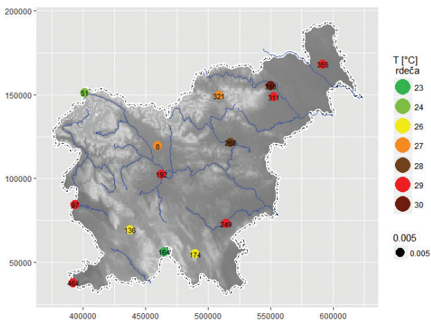
Slika 4. Enako kot slika 3, le za rdečo stopnjo ogroženosti. Figure 4. The same as figure 3, but for red level of threat.
