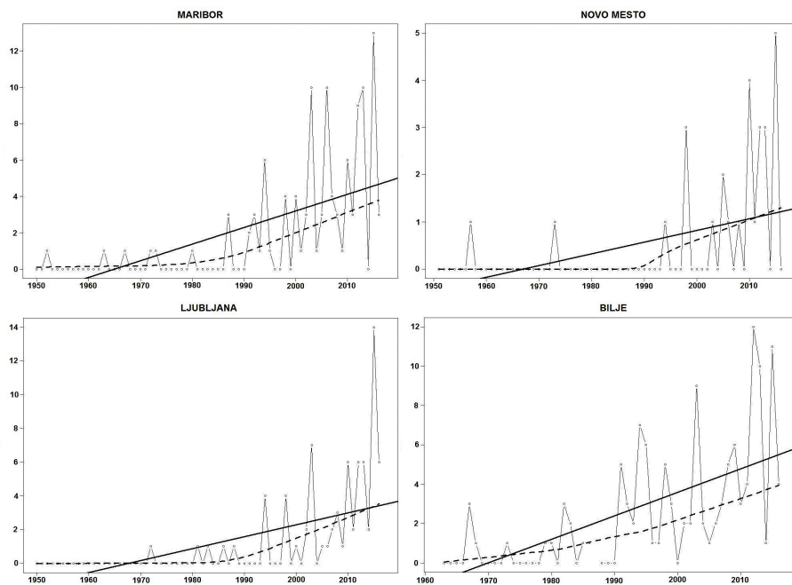
Slika 14. Prikaz števila tropskih noči na posameznih postajah v posameznih letih in njihov linearni trend naraščanja. Po vrsti so prikazane postaje Maribor, Novo mesto, Ljubljana in Bilje.
