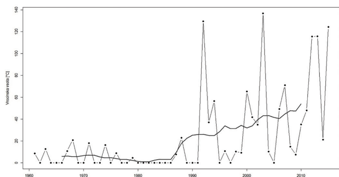
Slika 3. Vročinska vsota (-●-), ki je izračunana kot vsota odstopanj najvišjih dnevni temperatur zraka od praga 29,5 °C v vseh dneh v vročinskih valovih v posameznem letu, in desetletna drseča sredina (-) za obdobje 1961–2015 za Mursko Soboto.
