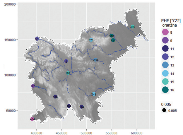
Slika 5. Vrednosti vročinskega kazalca EHF za oranžno stopnjo ogroženosti na posameznih obravnavanih postajah po Sloveniji. Številke na obarvanih krogih na zemljevidu predstavljajo številko postaje.
