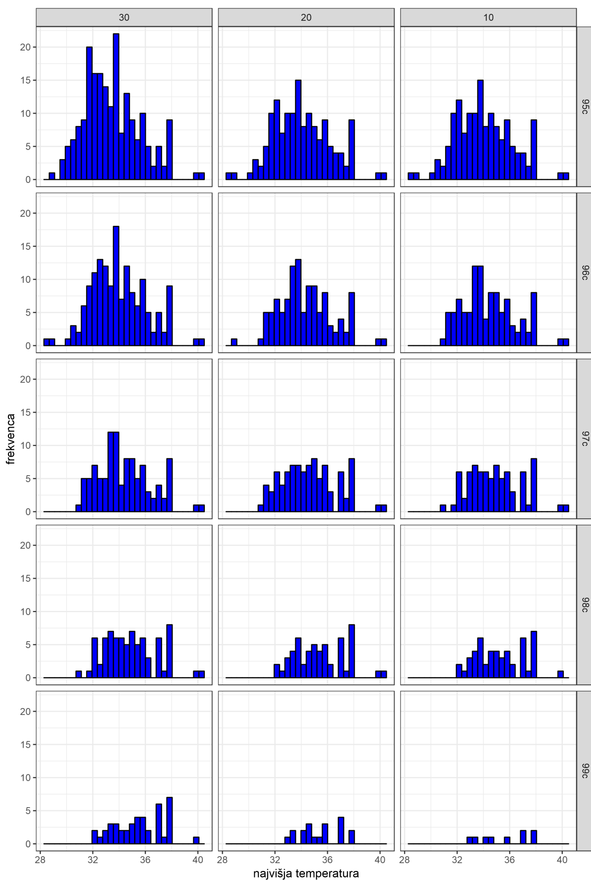
Slika 3. Porazdelitve dnevne najvišje temperature v času vročinskih valov na postaji v Črnomlju za vse obravnavane mejne vrednosti (različne centile in različna obdobja).
