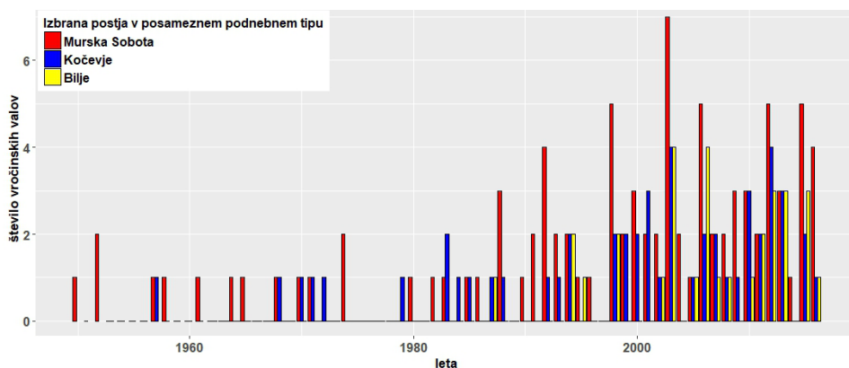
Slika 6. Število vročinskih valov na leto na postajah Murska Sobota (celinsko podnebje), Kočevje (zmerno podnebje hribovitega sveta) in Bilje (omiljeno sredozemsko podnebje).
