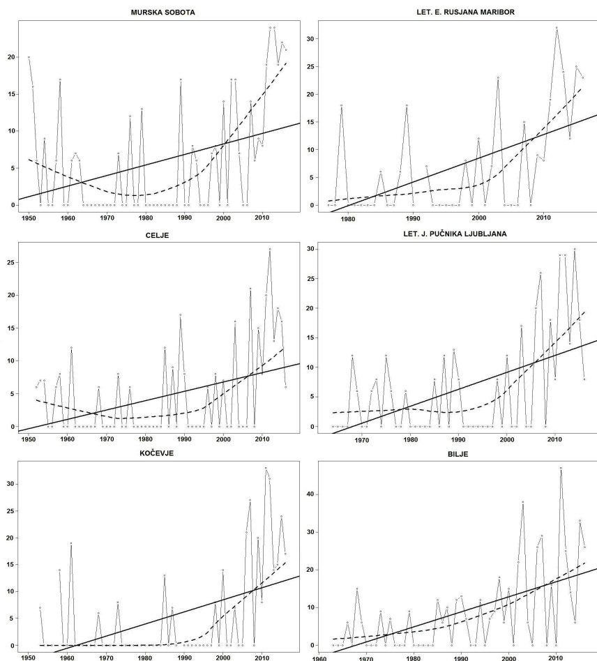
Slika 16. Enako kot slika 15 le da so tu prikazani rezultati kazalca trajanja vročinskega vala (WSDI) za postaje Murska Sobota, Letališče E. Rusjana Maribor, Celje, Let. J. Pučnika Ljubljana, Kočevje in Bilje.
