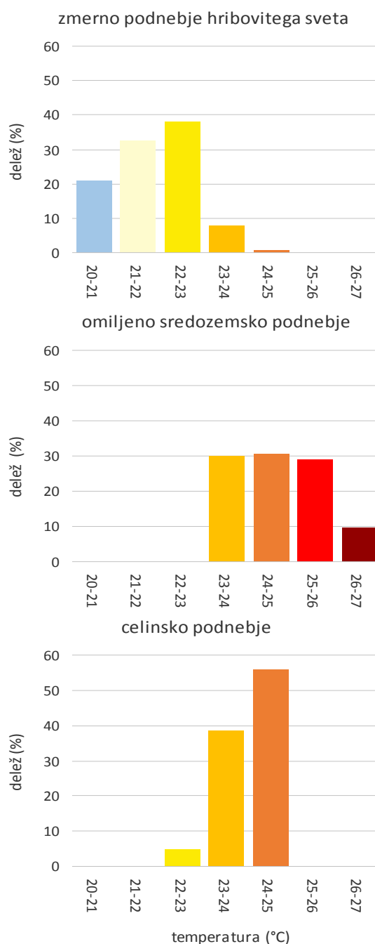
Slika 5.. Pogostost pojavljanja posameznih vrednosti DPT96 znotraj posamezne temperaturne regije. Frekvenčna porazdelitev za regijo z zmernim podnebjem hribovitega sveta je izračunana za celotno regijo, vključujoč območje z gorskim podnebjem.
