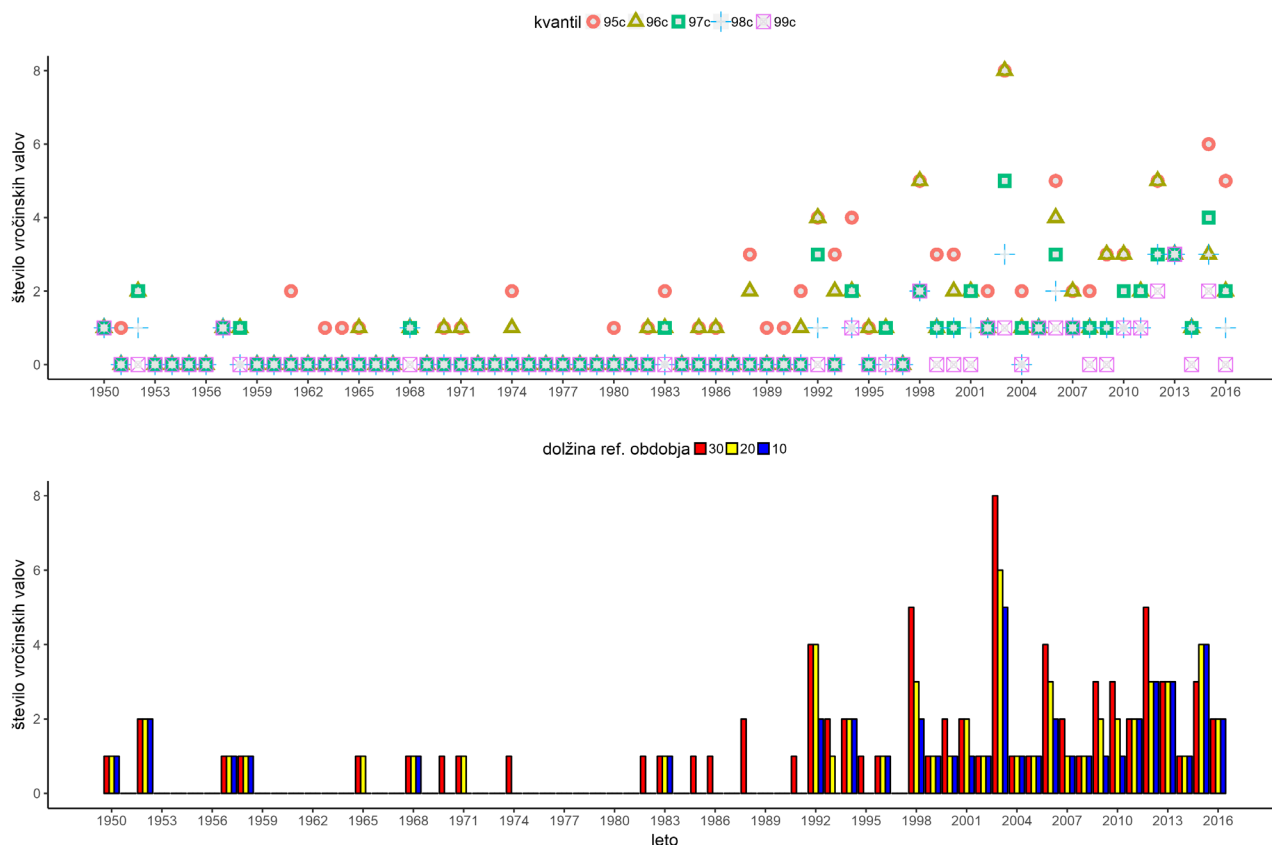
Slika 2. Število vročinskih valov na leto v Ljubljani v odvisnosti od izbire mejne vrednosti (zgoraj) in od izbire referenčnega obdobja (spodaj). Zgornja slika torej prikazuje število vročinskih valov za vseh pet mejnih vrednosti definiranih s centili, ki so izračunani s pomočjo najdaljšega referenčnega obdobja (1986-2015). Na spodnji sliki so prikazani rezultati za vsa tri referenčna obdobja, vendar samo za izbrani centil (96.). Zelene pike na zgornjem grafu tako predstavljajo iste vrednosti, kot rdeči stolpci na spodnjem grafu.
