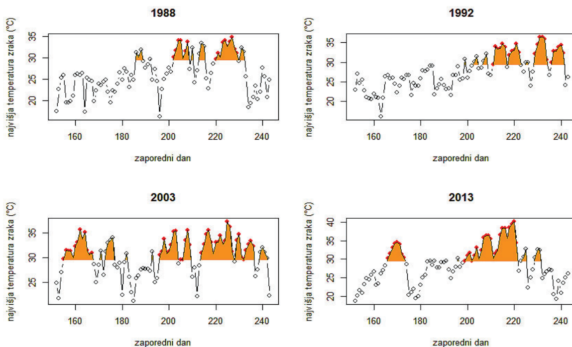
Slika 2. Vročinski valovi v Ljubljani v letih 1988, 1992, 2003 in 2013 – dnevi v vročinskih valovih so označeni z rdečo, vsi dnevi nad pragom 29,5 °C pa so označeni z oranžnim območjem (160. dan = 9. junij, 240. dan = 28. avgust) (Zalar in sod. 2017).
