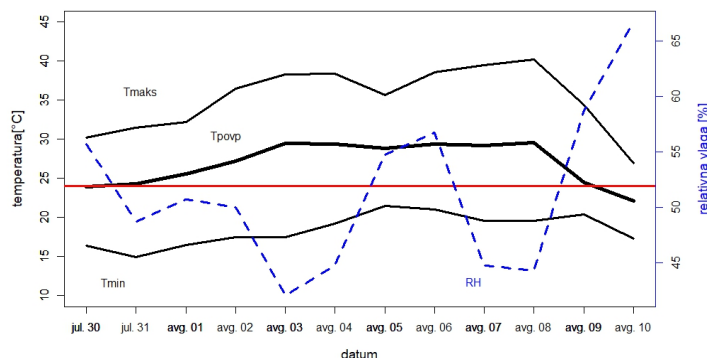
Slika 7. Potek dnevne najvišje, najnižje in povprečne temperature ter relativne vlažnosti v vročinskem valu ob koncu julija in začetku avgusta 2013 v Ljubljani. Z rdečo črto je označena mejna vrednost za vročinski val (glej preglednico 3). Dnevna povprečna temperatura je takrat mejo prekoračila kar v desetih zaporednih dneh.
