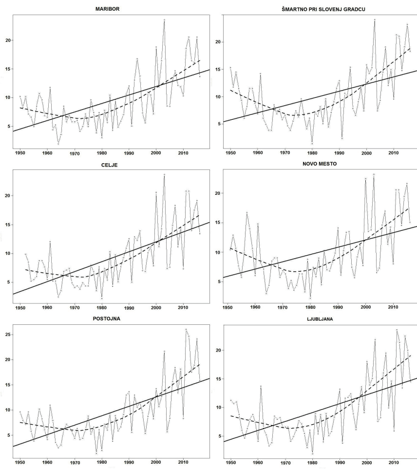
Slika 15. Prikaz deleža dni na leto, ko imamo preseženo mejo 90 percentila najvišjih dnevnih temperatur s pet dnevni oknom izmerjenih na isti dan v letu v 30 letnem referenčnem obdobju. Po vrsti so tokrat predstavljene postaje: Maribor, Šmartno pri Slovenj Gradcu, Celje, Novo mesto, Postojna in Ljubljana.
