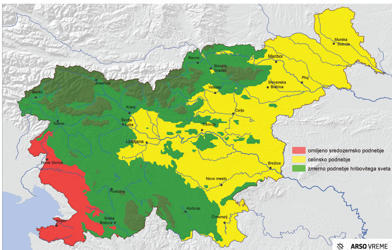
Slika 1. Temperaturne regije, povzete po Kozjek in sod. (2016), namenjene analizi vročinskih valov. Temno območje znotraj regije s podnebjem hribovitega sveta (zelena), predstavlja območje z gorskim podnebjem, ki ni bilo vključeno v analizo.
