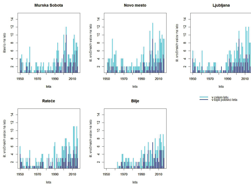
Slika 10. Prikaz števila vročinskih valov po definiciji iz kazalca HWMID. Vsi vročinski valovi v letu, torej tudi zimski, so prikazani s turkizno barvo, samo tiste v toplejši polovici leta prikazujejo modri stolpci. Po vrsti so prikazane postaje Murska Sobota, Novo mesto, Ljubljana, Rateče in Bilje.
