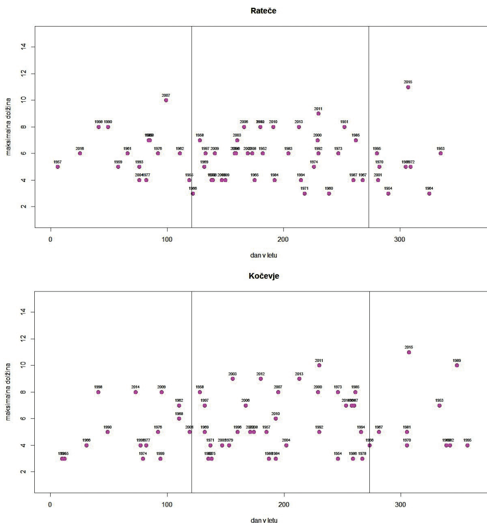
Slika 12. Enako kot slika 11, le da sta tu predstavljeni postaji Rateče in Kočevje, ki sta imeli absolutno najdaljši vročinski val v hladni polovici leta 2015.
