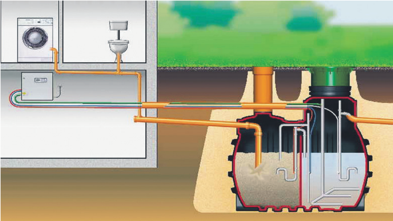
Primer delovanja male komunalne čistilne naprave (vir: www.adut.si )
