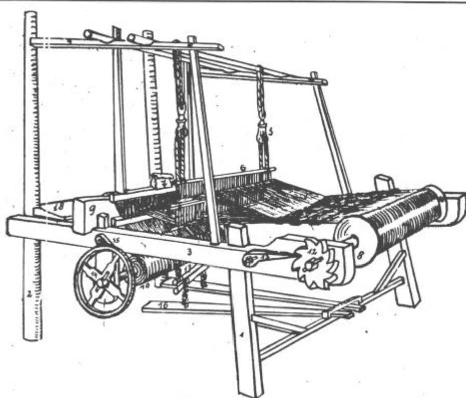
Sokatnikove statve, Gornji grad št. 119 (shematična risba). Legenda: 1 koza, 2 navpična stebrašča, 3 ojnica, 4 ostršeje, 5 knobe, 6 grebeni, 7 žlage, 8 prvi pom s šajooma, 9 zadnji pom, 10 spodnji pom, 11 šajba, 12 oven, 13 rigl, 14 kolo za špananje, 15 rigl na kolesu za špananje, 16 podnožjak ali nogavica, 17 vage, 18 klop.
