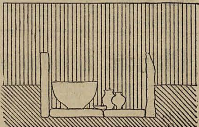
Prerez skozi rimski grob v Rojah pri Šentjerneju
