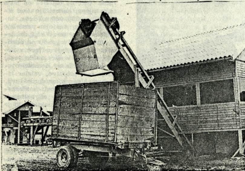
Rešitev za odvoz lubja na central. skladišču v Pivki pri Postojni
