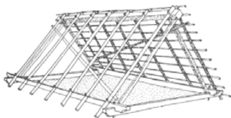
Preprosta strešna konstrukcija s slemenskim tramom
