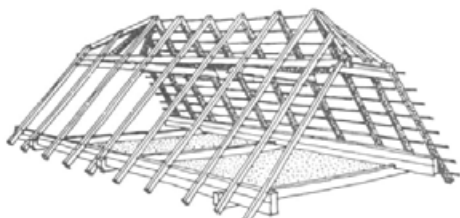
Konstrukcija čopaste dvokapnice z vmesnimi legami in škarjami
