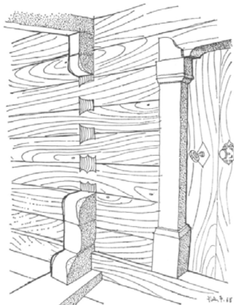
Detajl konstrukcije stene in portala — Loke v Tuh. dolini
