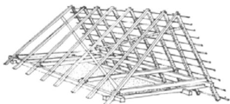
Dvokapnica brez vmesnih leg in s škarjastimi vezmi
