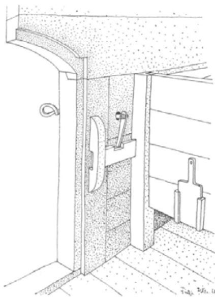
Detajl vratne »ključavnice« in predelov — Mali hrib 10
