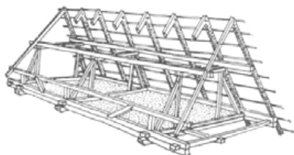
Nesimetrična dvokapnica z nosilnim ogrodjem — trapeznim razpiralom
