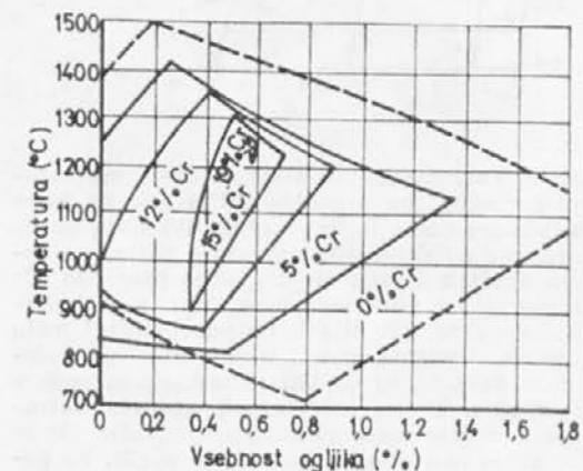
Sl. 5. Pri katerih temperaturah in kakih vsebnostih ogljika ter kroma se pojavlja gama faza (avstenit).
