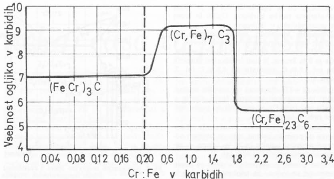
Sl. 2. Količina ogljika, kroma in železa v različnih tipih karbidov (kemijskih spojin kovin z ogljikom).
