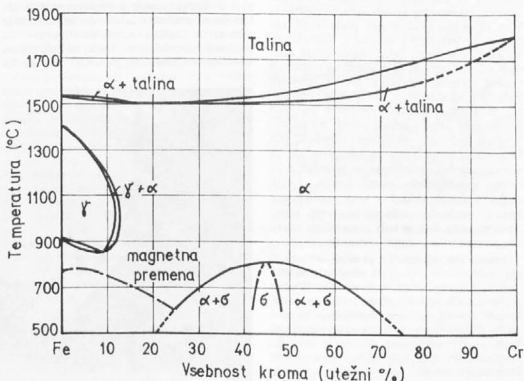
Sl. 1. Strukture Fe — Cr zlitin pri različnih temperaturah.
