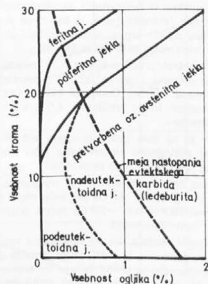
Sl. 8. Kombinacije vsebnosti ogljika in kroma, ki opredeljujejo vrste jekla (strukturo) pri navadni temperaturi.
