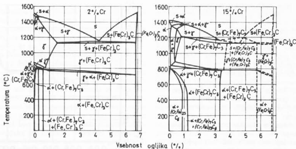
Sl. 7. Strukturne sestavine jekel z različnimi vsebnostmi ogljika in z 2 ali 15 % kroma pri različnih temperaturah. Prereza skozi ternarni sistem Fe-CR-C.
