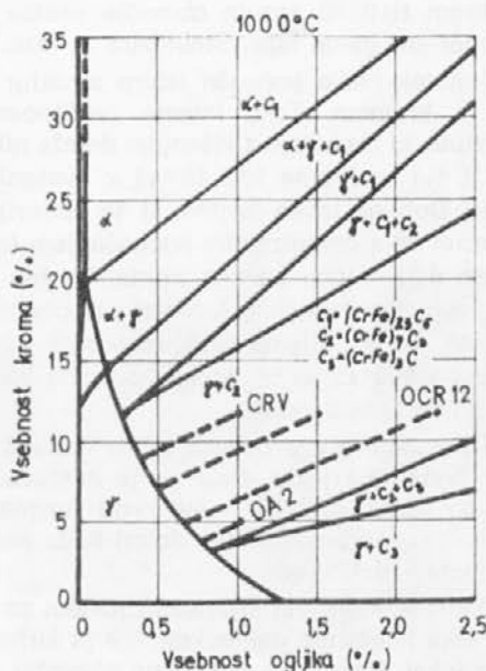
Sl. 3. Vrste struktur jekla pri 1000° C v odvisnosti od vsebnosti ogljika in kroma v jeklu.
