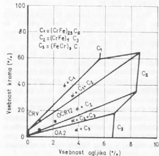
Sl. 4. Vrste struktur pri 700° C v odvisnosti od vsebnosti ogljika in kroma v jeklu.
