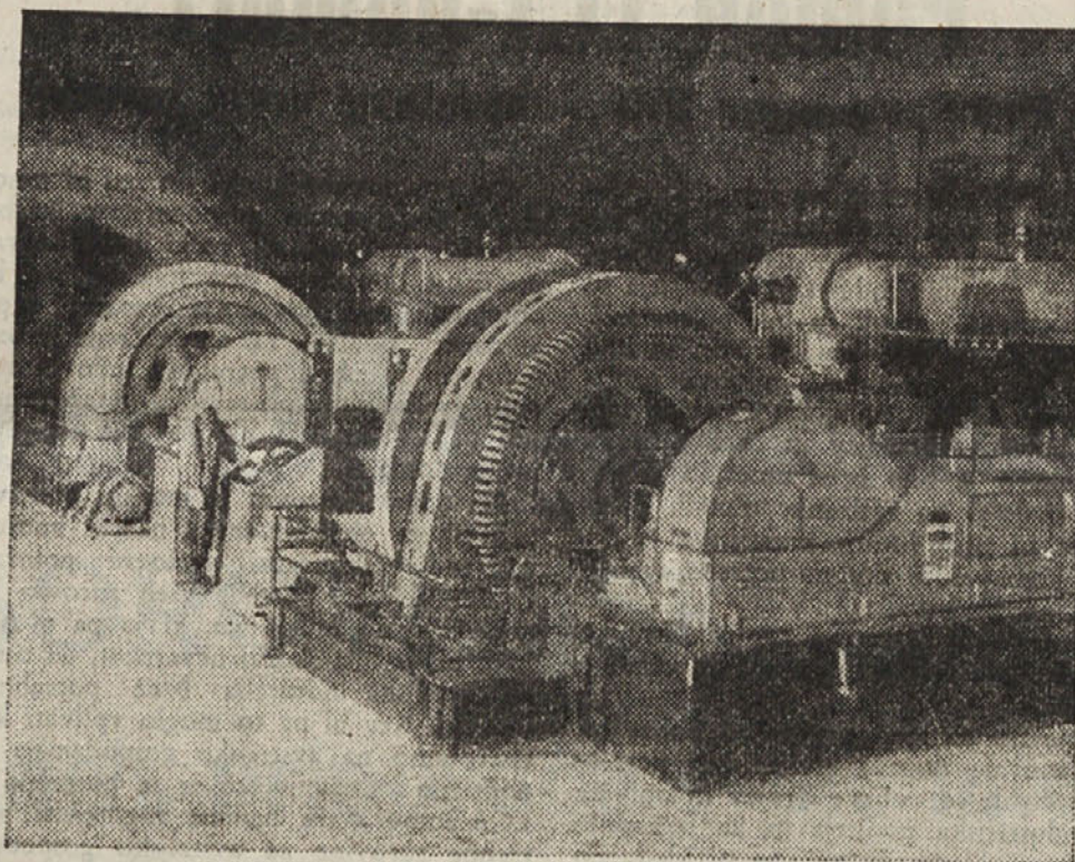
Jeklarnam Donawitz je ERP-pomoč dobavila iz Amerike poleg drugih strojev tudi horizontalni batni kompresor (Kolbenkompressor) za 700 konjskih sil. Novi stroji bodo omogočili povečanje proizvodnje jekla in železa že letos za 25 odstotkov.
