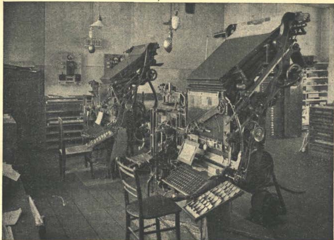
Stavna stroja linotajpa v tiskarni v Celju.
