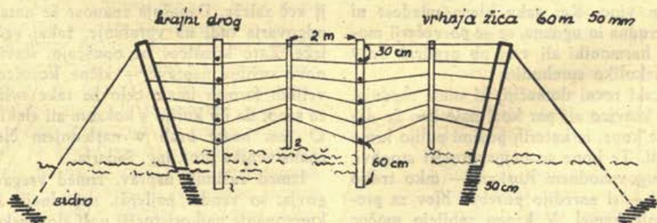
Žični kozolec od strani.
