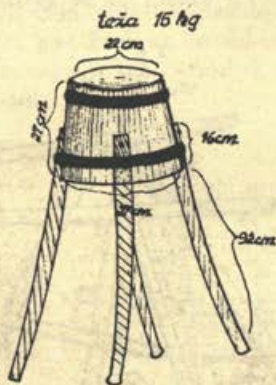
Zabijač, opasan z železnima, 3 cm širokima in 3 mm debelima obročema. Dva delavca ga dvigata in spuščata na kol, ki ga drži in uravnava tretji delavec.
