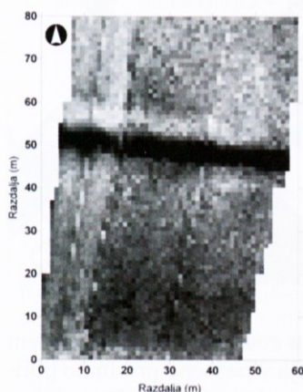
Slika 3: Odsek ceste Neviodunum - Siscia v Veliki dolini med Ribnico in Podgračnim na rezultatih geoelektričnega kartiranja.
