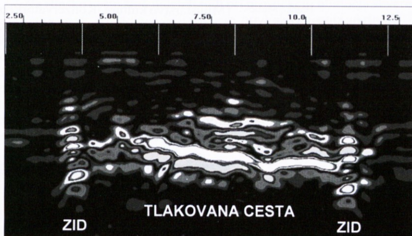
Slika 2: Vrhnika ( Nauportus ). Georadarski profil čez tlakovano cesto (glej sliko 1). Lepo se vidijo izraziti odboji od »horizontalne plasti«, ki je v tem primeru s kamnitimi ploščami tlakovana cesta.
