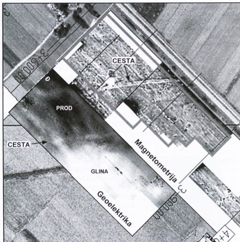
Slika 4: Velika Gorica – Gradiči. Primerjava rezultatov magnetne in geoelektrične metode na eni od južnih vpadnic Andautonije. Na prodnato-peščeni podlagi se isti odsek ceste kaže kot pas nizkih vrednosti električne upornosti.
