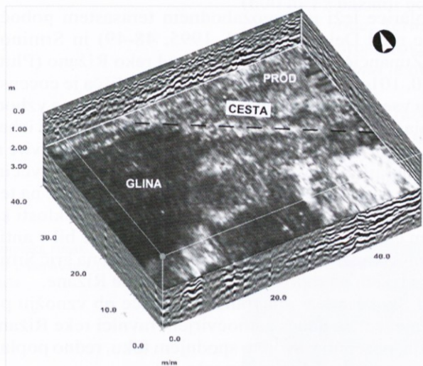
Slika 5: Velika Gorica – Gradiči. Tridimenzionalen prikaz georadarskih odbojev na območju, kjer je bila cesta ugotovljena z magnetno in geoelektrično metodo (slika 4).
