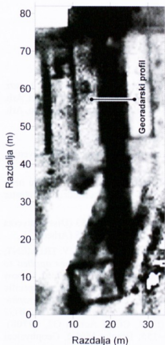
Slika 1: Vrhnika ( Nauportus ). Širok pas visokih vrednosti upornosti v smeri sever – jug je posledica tlakovane ceste, ki povezuje breg Ljubljaničnice s centralnim delom antičnega kompleksa. Označen je položaj georadarskega profila, ki je prikazan na sliki 2.
