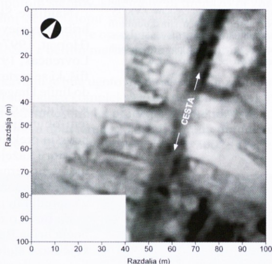
Slika 6: Ščitarjevo – Andautonia. Severna vpadnica v Andautonio na rezultatih geoelektričnega kartiranja.
