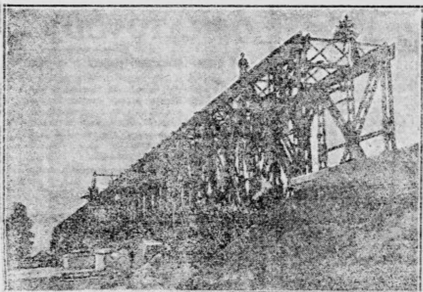
Veliki železniški most čez Muro pri Veržeju.
