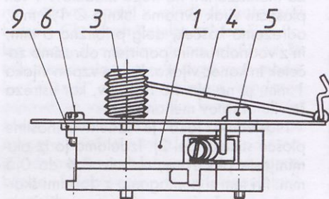
Risba 1. Delovanje determalnega sistema
