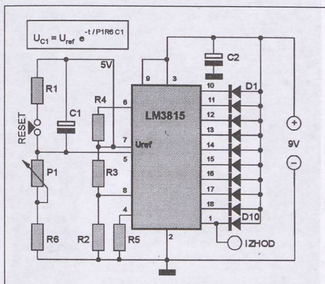
Shema vezja
