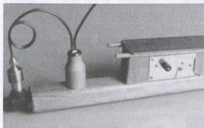
Slika 4. CO 2 -model s časovnim stikalom
