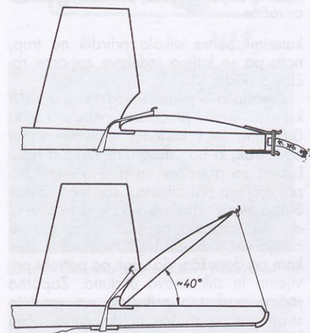
Risba 1. Delovanje determalnega sistema
