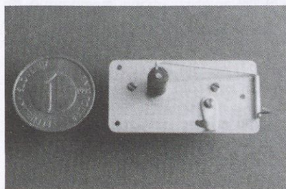
Slika 3. Časovno stikalo TOMY in kovanec za 1 SIT
