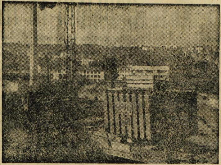
Transport transformatorja 8000 KVh za novo razdelilno postajo Zlato polje
