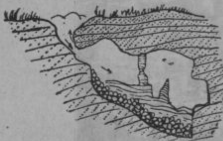
Risba 18.: Prerez Beilsteinhöhle (po Bocku).
