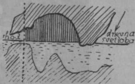
Risba 19.: Prerez biševske jame (V. Bohinec).
