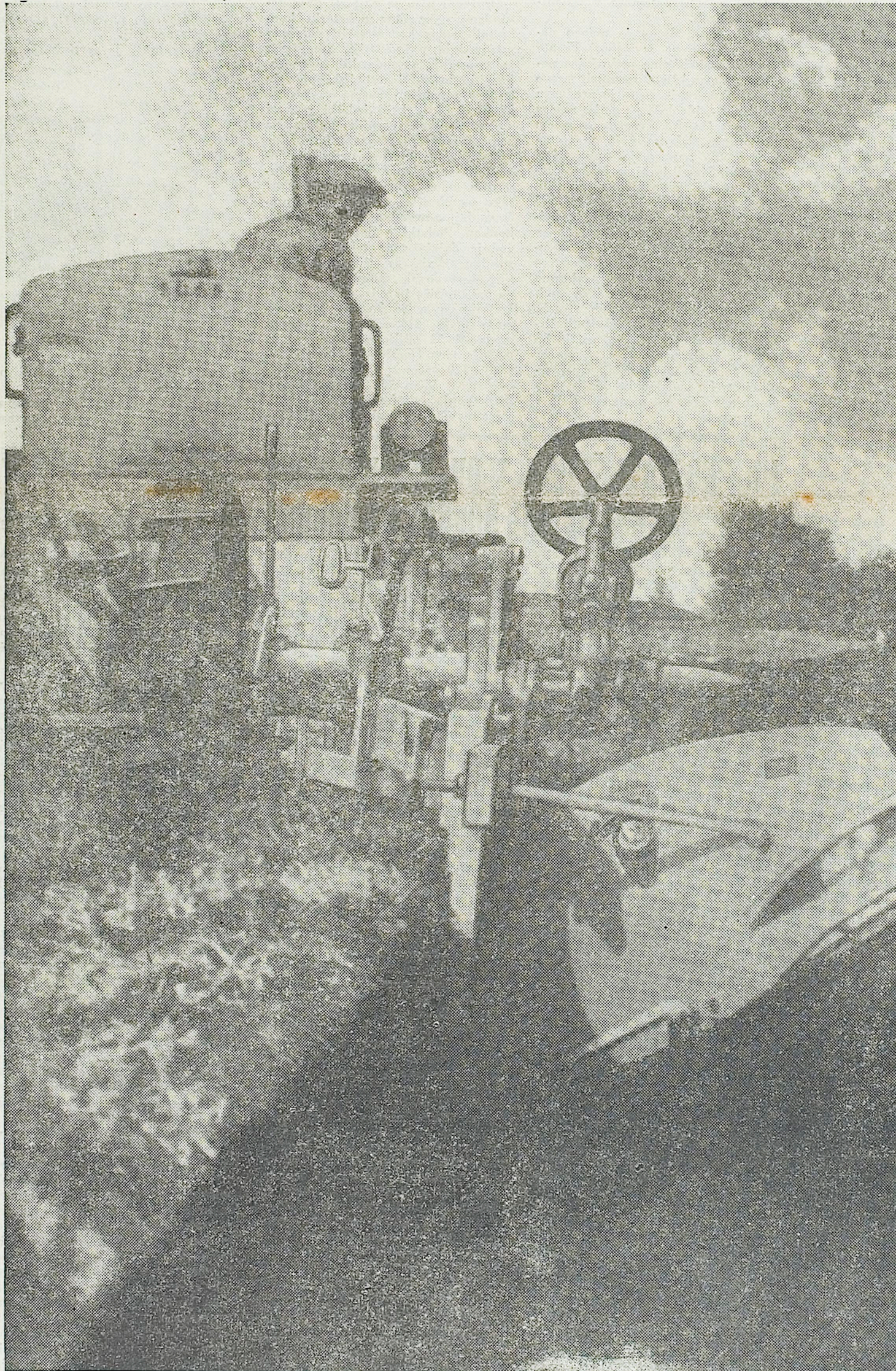
SKLAD ZA MEHANIZACIJO PRI OKRAJNI ZADRUŽNI POSLOVNI ZVEZI V KOPRU JE NABAVIL VEČ TEŽKIH TRAKTORJEV ZA RIGOLANJE VINOGRADOV IN JIH PORAZDELIL KMEČKIM DELOVNIM ZADRUGAM. NA SLIKI VIDIMO TRAKTOR ANSALDO 60 S KAKRSNIM SO ZADRUGAM ZNANI IZ PUČ-KOŠTADONE PREORALI VELIK KOMPLEKS ZEMLJIŠČA V BRIČU
