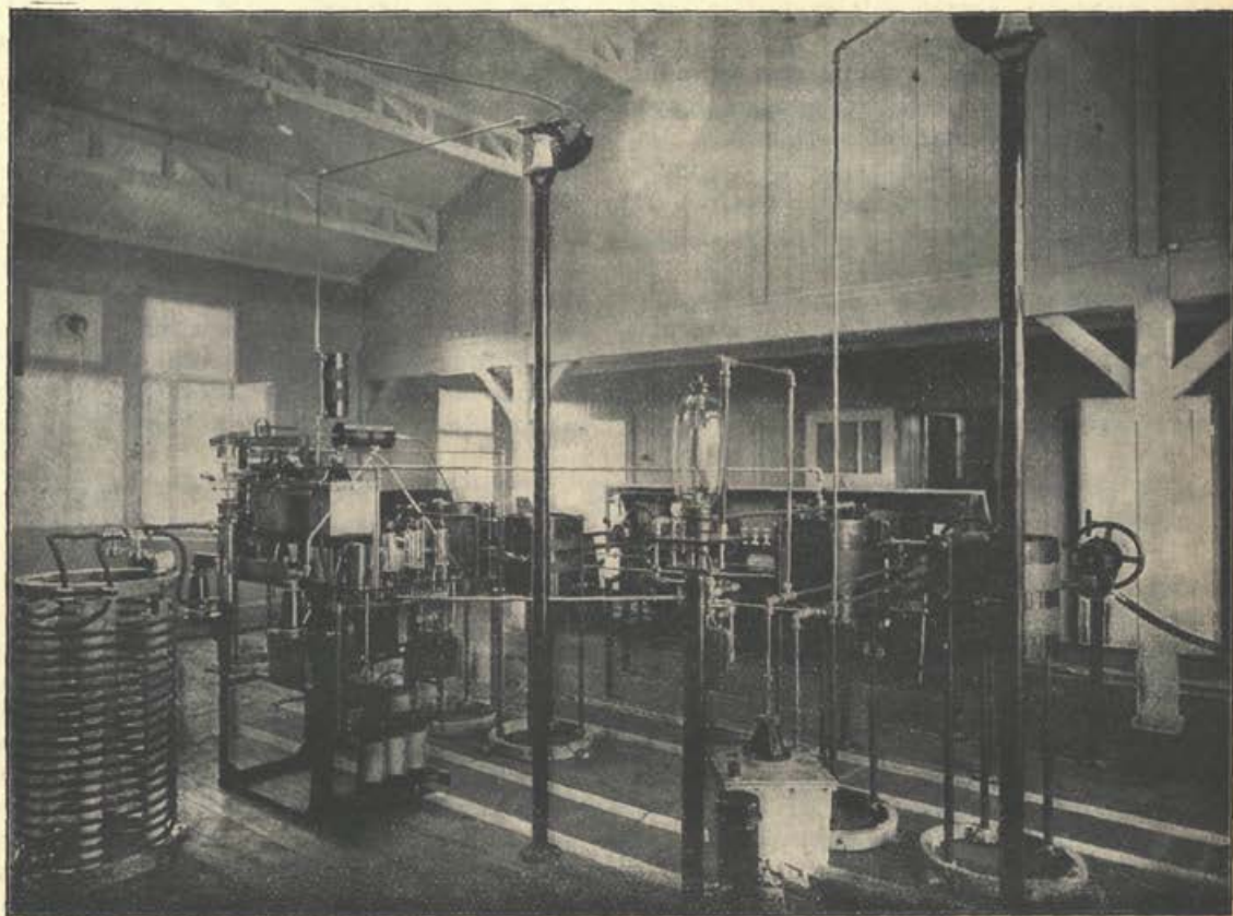
Glavni oddajni aparati. (Priprave za vzbujanje in odpošiljanje valov-radio.)
