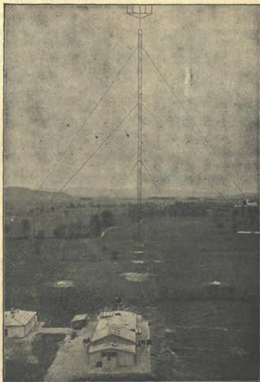
Pogled na radio-postajo v Domžalah z aeroplana. Dobro je videti velikansko anteno.
