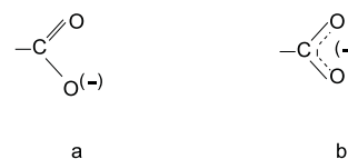
Slika 2: Delokalizirana struktura pri nastanku soli: a) struktura z lokalizirano vezjo \text{C=O} ; b) simetrično ionizirana struktura
