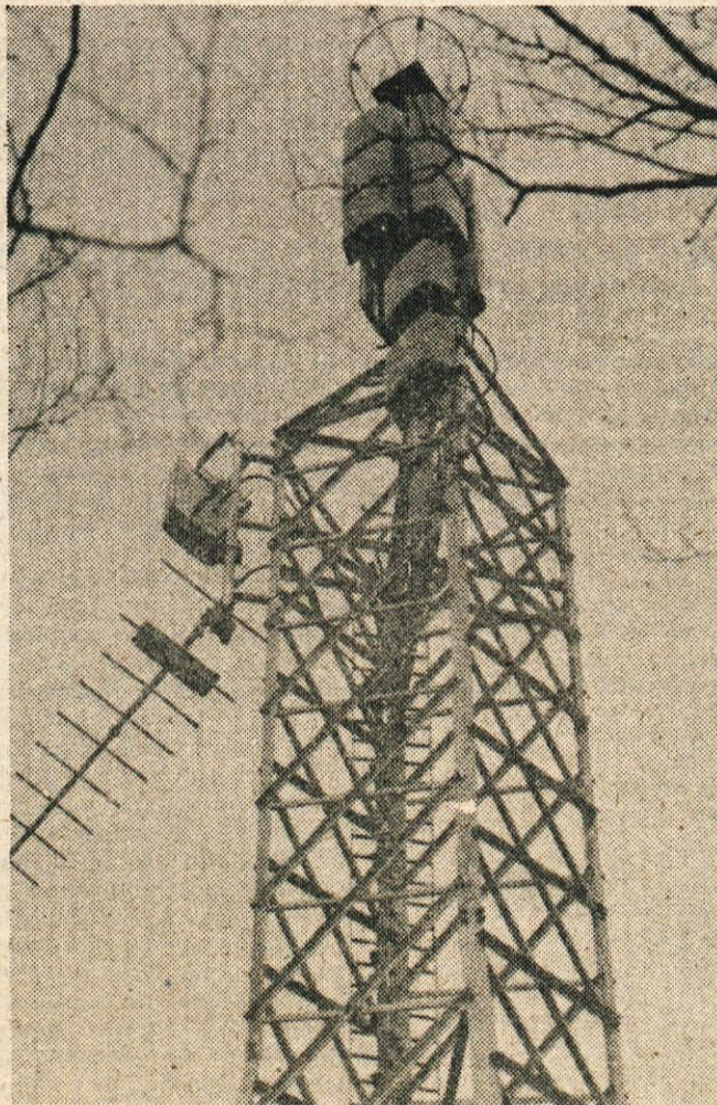
Sprejemno oddajne naprave na pretvorniku Gorišca
