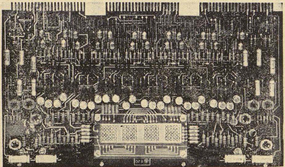
Posnetek prikazuje enoto elektronske fakturirke s feritnim pomnilnikom
