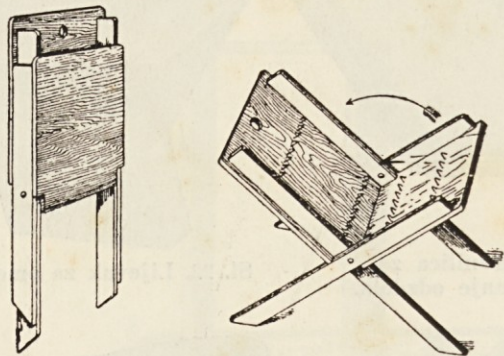
Sl. 24. Zaklopni kozlić otvoren i zatvoren.
