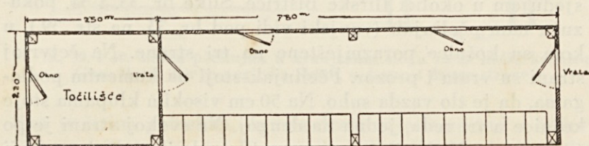
Sl. 36. Tloris jednostranog pčelinjaka sa vrcalištem za 54 naših košnica. Po ovom nacrtu je izgrađen moj vanjski pčelinjak u Ribnici kod Ilirske Bistrice. (Najpraktičniji oblik pčelinjaka.)
