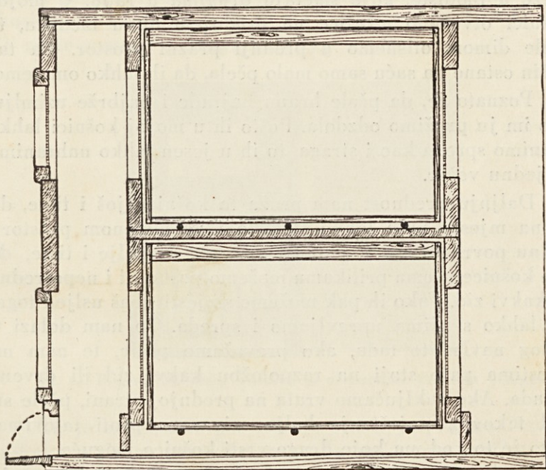
Sl. 13. Prema mojem izumu usavršena košnica. Prerez po dužini.
