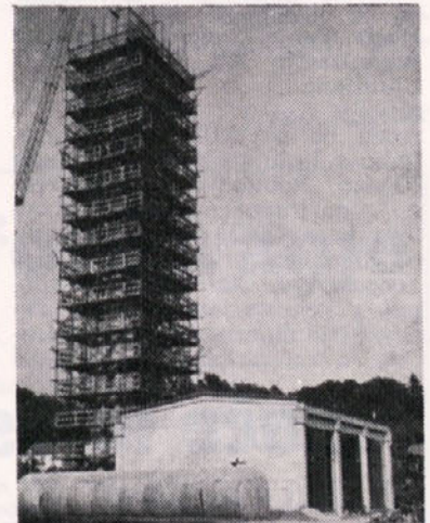
Centralna kotlarna v Ratanjski vasi, zgrajena po našem montažnem sistemu
