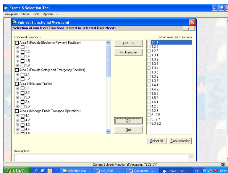
Slika 7: Izbira osnovnih funkcij glede na izbrane potrebe uporabnikov
