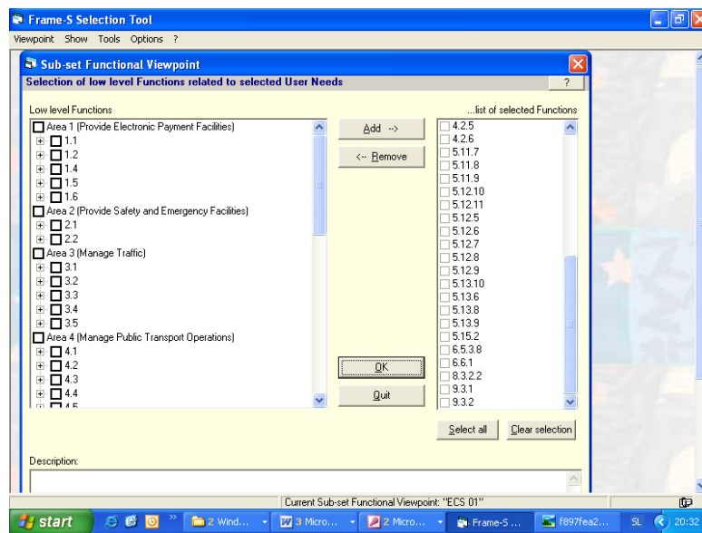
Slika 16: Izbira osnovnih funkcij glede na izbrane potrebe uporabnikov
