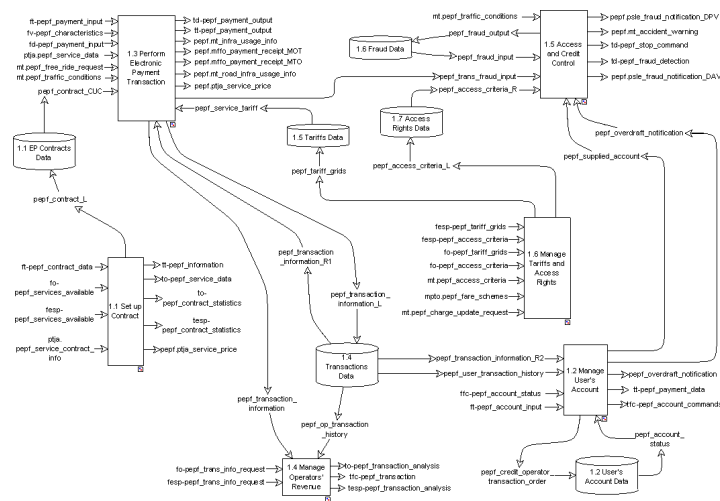
Slika 5: Shematski prikaz funkcije »Perform Electronic Payment Transaction«
