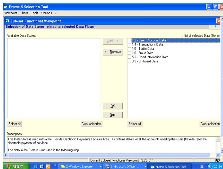
Slika 18: Izбира podatkovnih skladišč glede na izbrane tokove podatkov
