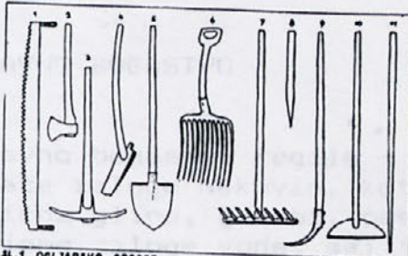
SL.1 OGLJARSKO ORODJE 1 ŽAGA, 2 ŠERHAR, 3 ŠERHAR, 4 POKAL, 5 KOPAL, 6 VILJ, 7 ŠERHARJE, 8 LUKANJE, 9 KALINA, 10 OROBLJAK, 11 BOHANČICA
