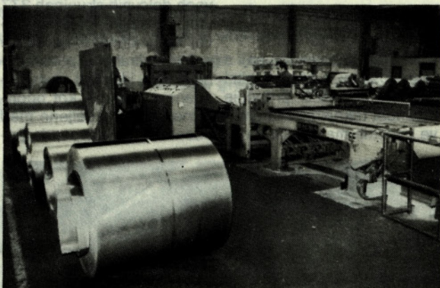
TOZD POSODA – surovinski obrat – stroj za razrez colsov.
