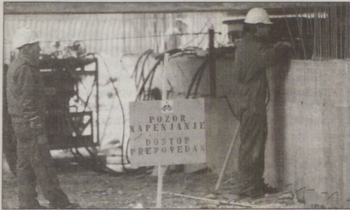
Tehnika narivne gradnje je novost v slovenskem gradbeništvu.
