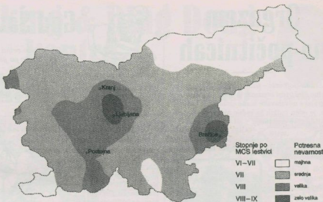
12- stopenjska opisna potresna lestvica MSK, MCS, EMS (Mercallijeva lestvica)
