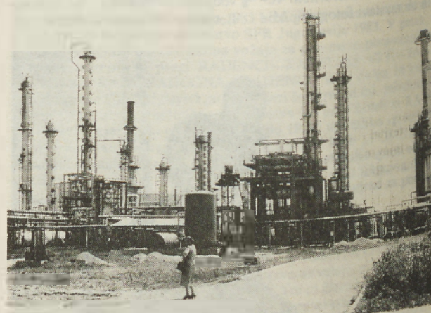
Pogled na del rafinerije INA-NAFTA Lendava.
