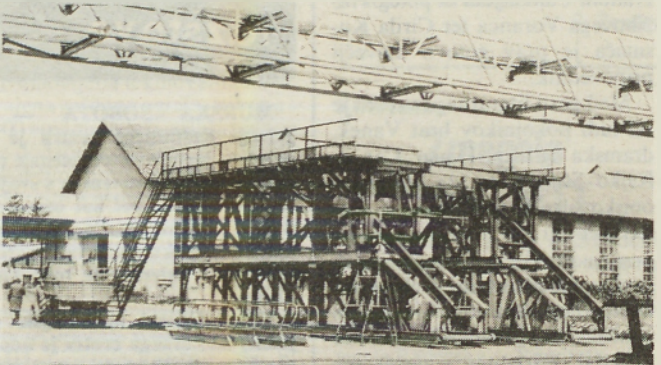
Gradnja vrtnega stolpa v tozd STROJNE DELAVNICE.
