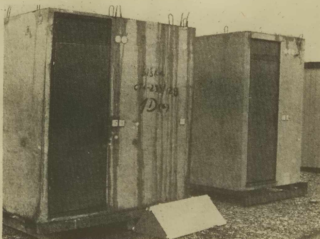
– Sanitarne kabine za industrijsko izgradnjo stanovanj – Gorenje Varstroj Lendava
