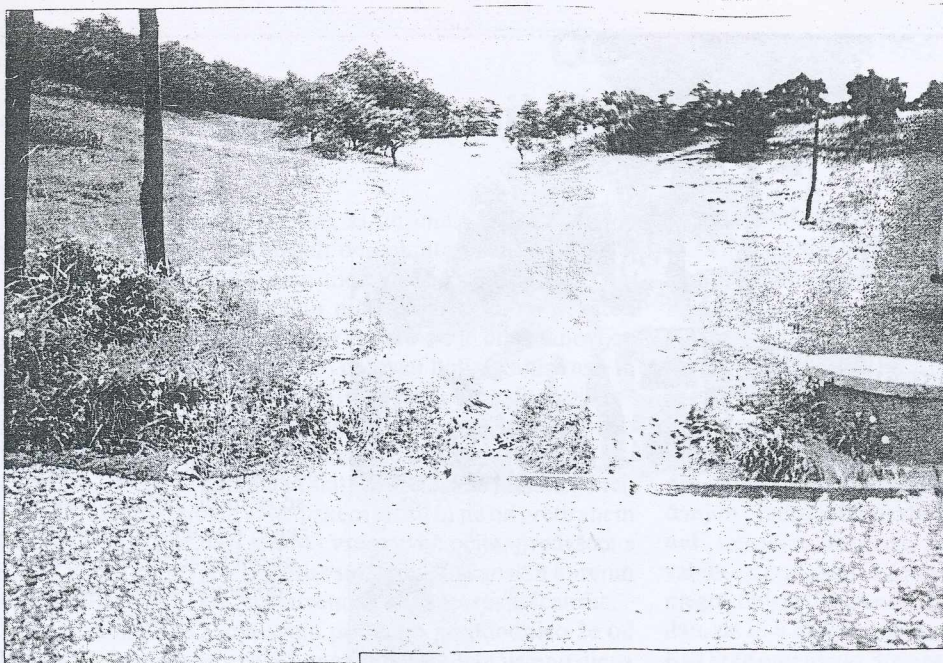
Sanacija plazu v Stanjevcih. Tudi po sanaciji se je pokazalo, da ogromne količine vode kljub sanaciji lahko poškodujejo teren, kar je dokaz, da je takšne objekte tudi potrebno vzdrževati.
