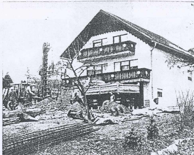
Priprava za betoniranje pilotov na plazu na domačiji Sukič, boreča 20.
