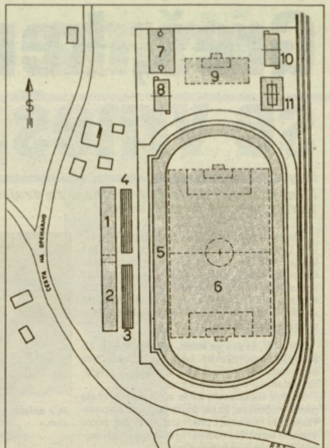
Načrt Olimpijskega stadiona iz leta 1958 s tribunami, atletsko stezo, dvorano, štiristeznim kegljiščem in igrišči za košarko, odbojko in posebnim prostorom za vadbo vratarjev.
