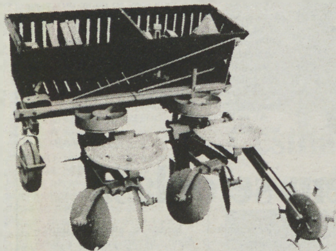
Sadilnik za krompir, polavtomatski, SK-2
