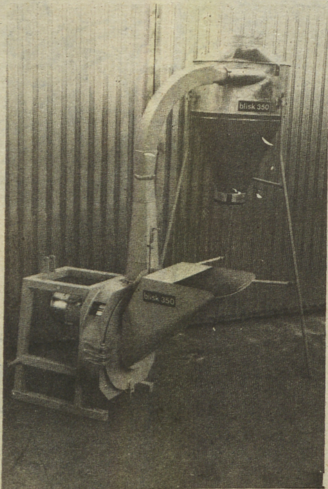
Drobilec za siliranje kornu v zrnu in storžih kapacitete: 2 t/h B 200 E, 8 t/h B 350 S in 15 t/h B 500 S. Vlažnost zrna do 40 odstotkov, višina transporta do 10 m.
