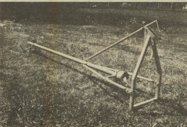
Mešalec gnojevke MGS, kapaciteta 15000 litrov-na uro, pogonska moč 15 kw.
