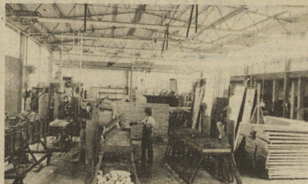
— V novih proizvodnih prostorih. Izdelovanje elementov in vrat za montažne hladilnice in komore.
