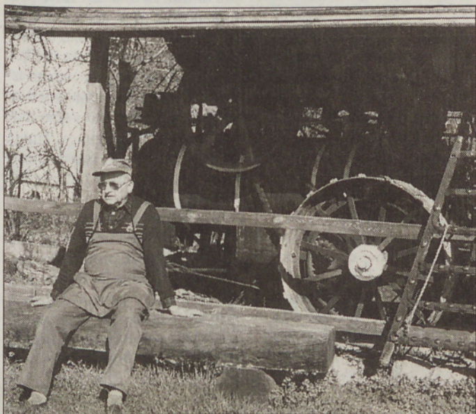
74 let stara lokomobila z lastnikom Antonom Kousom.
